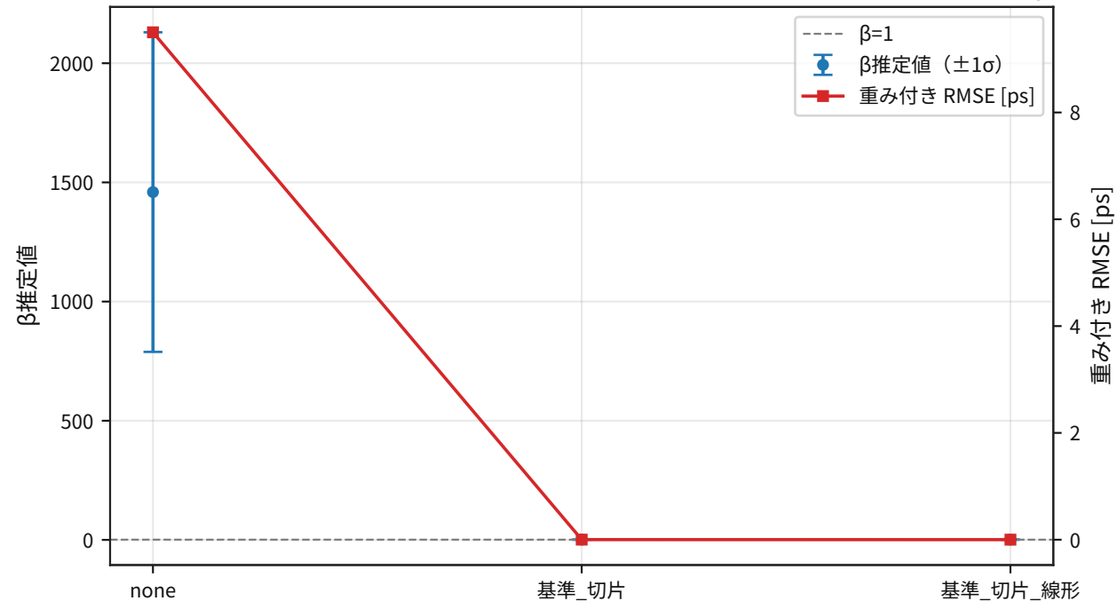
VLBI \beta 直接フィットの擾乱感度
