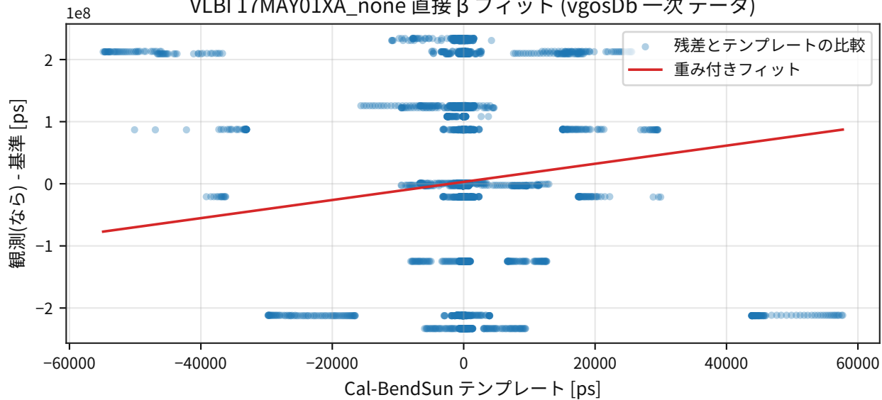
VLBI 17MAY01XA_none 直接 \beta フィット (vgosDb 一次 データ)
