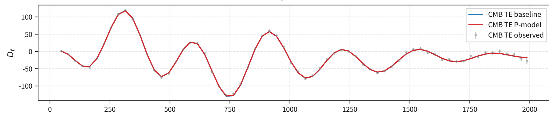
CMB TE
