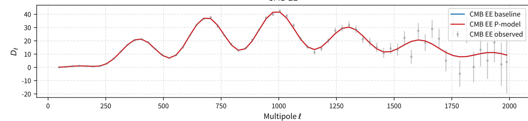
CMB EE
