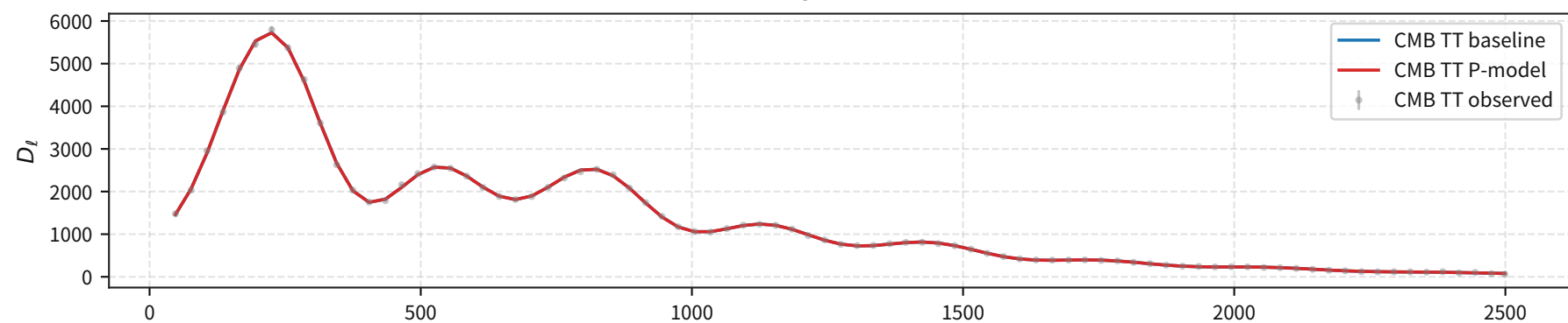
CMB TT
