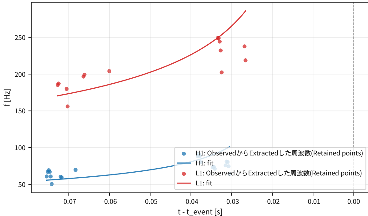
GW150914: 周波数 上る(chirp)様子 and 単純model 一致
