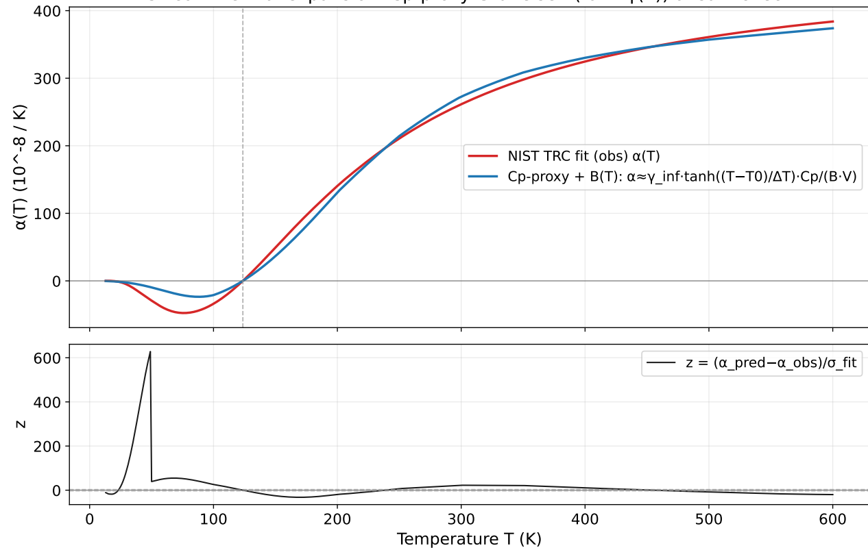
Silicon thermal expansion: Cp-proxy Grüneisen (tanh \gamma(T) ) ansatz check
