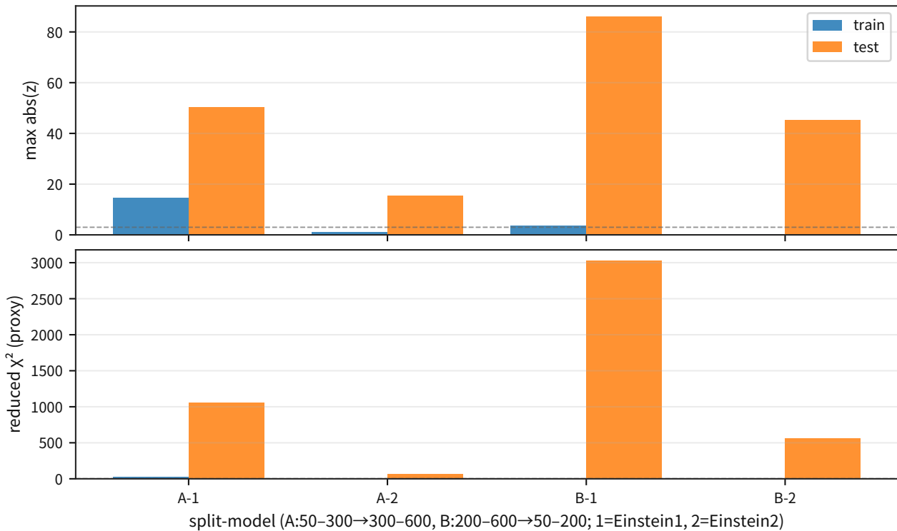
Si \alpha(T) : 温度分割 ホールドアウト (Debye+Einstein)
