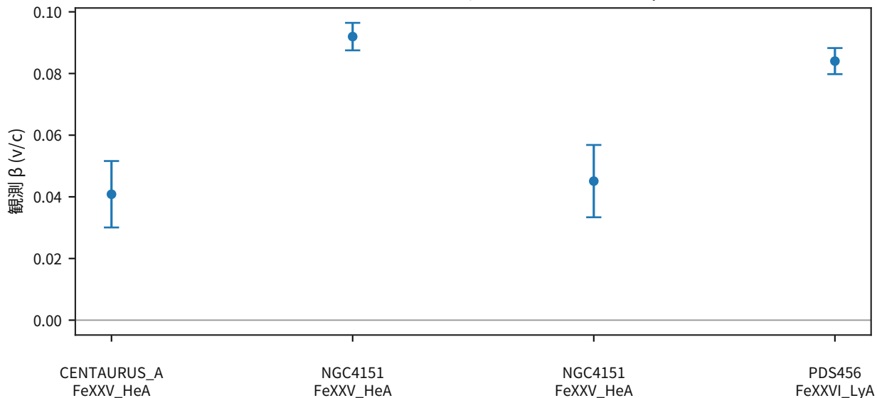
XRISM Resolve : BH/AGN 線重心からの \beta
