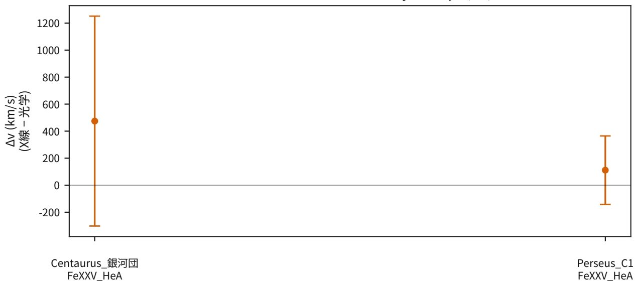
XRISM Resolve : 銀河団 z_{\text{xray}} - z_{\text{opt}} ( \Delta v )
