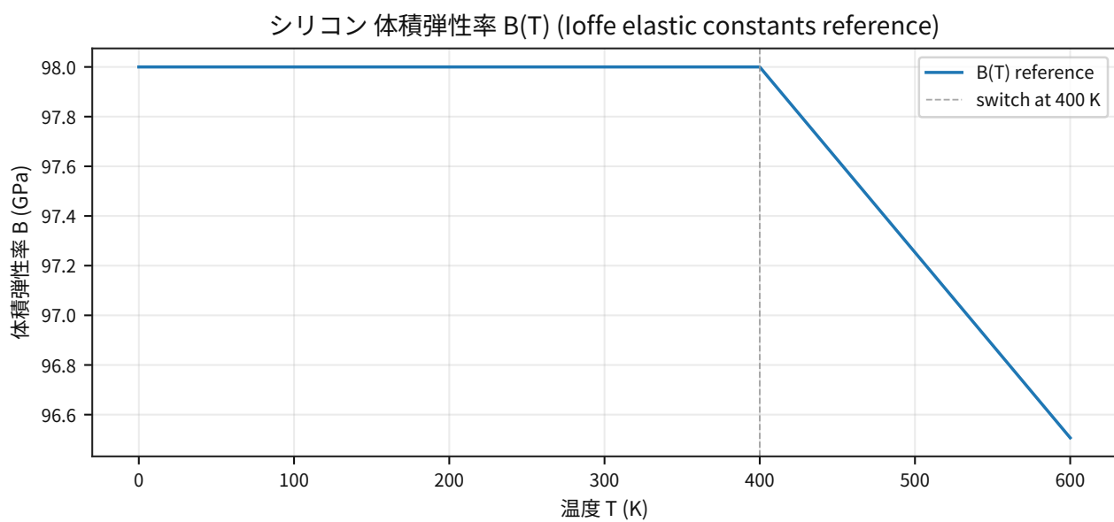
図 68: Ioffe の弾性定数から構成した B(T) を、切り分け用の独立入力として固定する。
