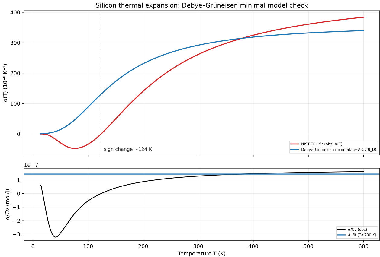
図 49: 上: \alpha(T) (一次固定) と、Debye – Grüneisen 最小モデル ( \alpha \approx A \cdot Cv ) の比較。
