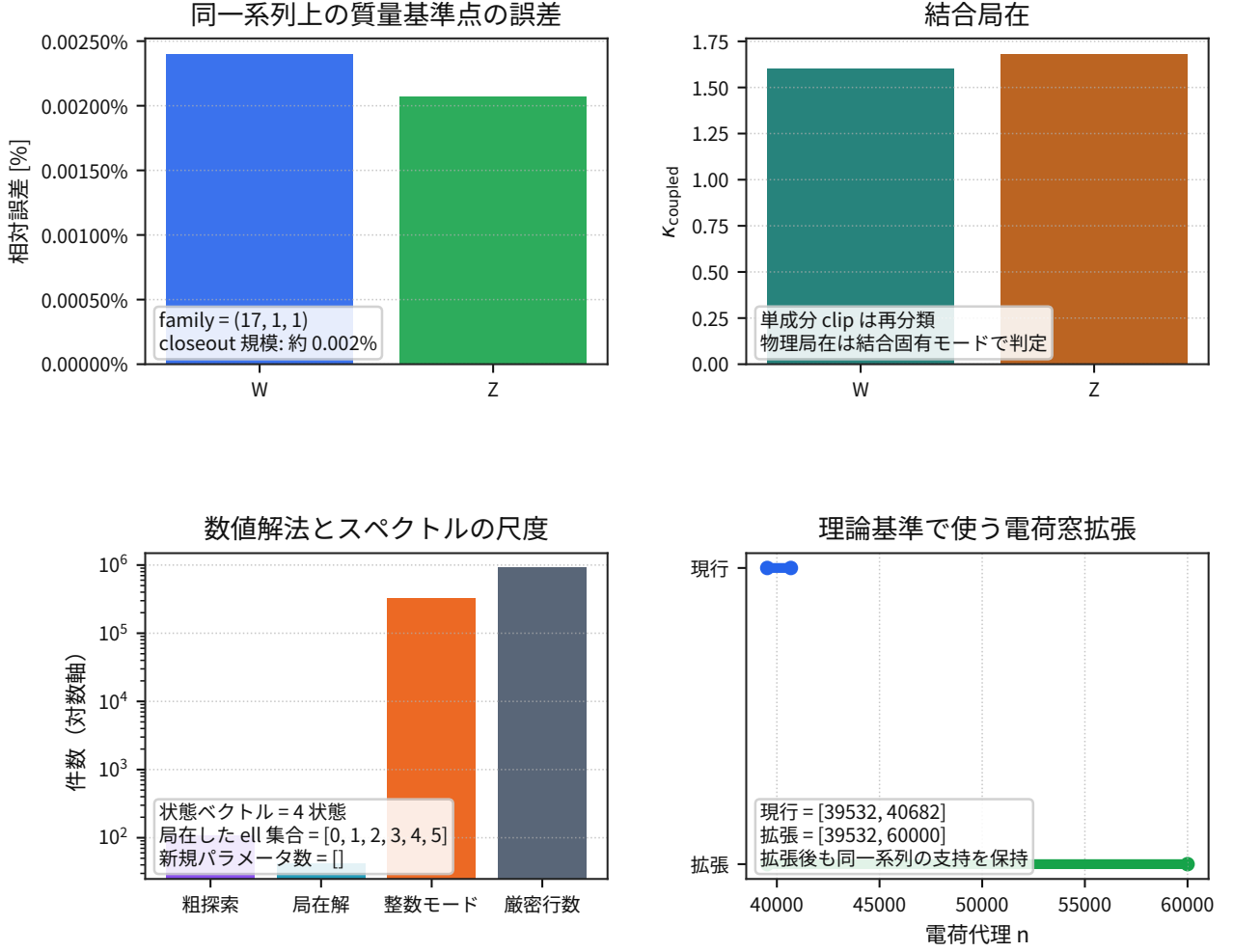
図 62: W/Z 質量基準点の結合局在条件による理論基準
