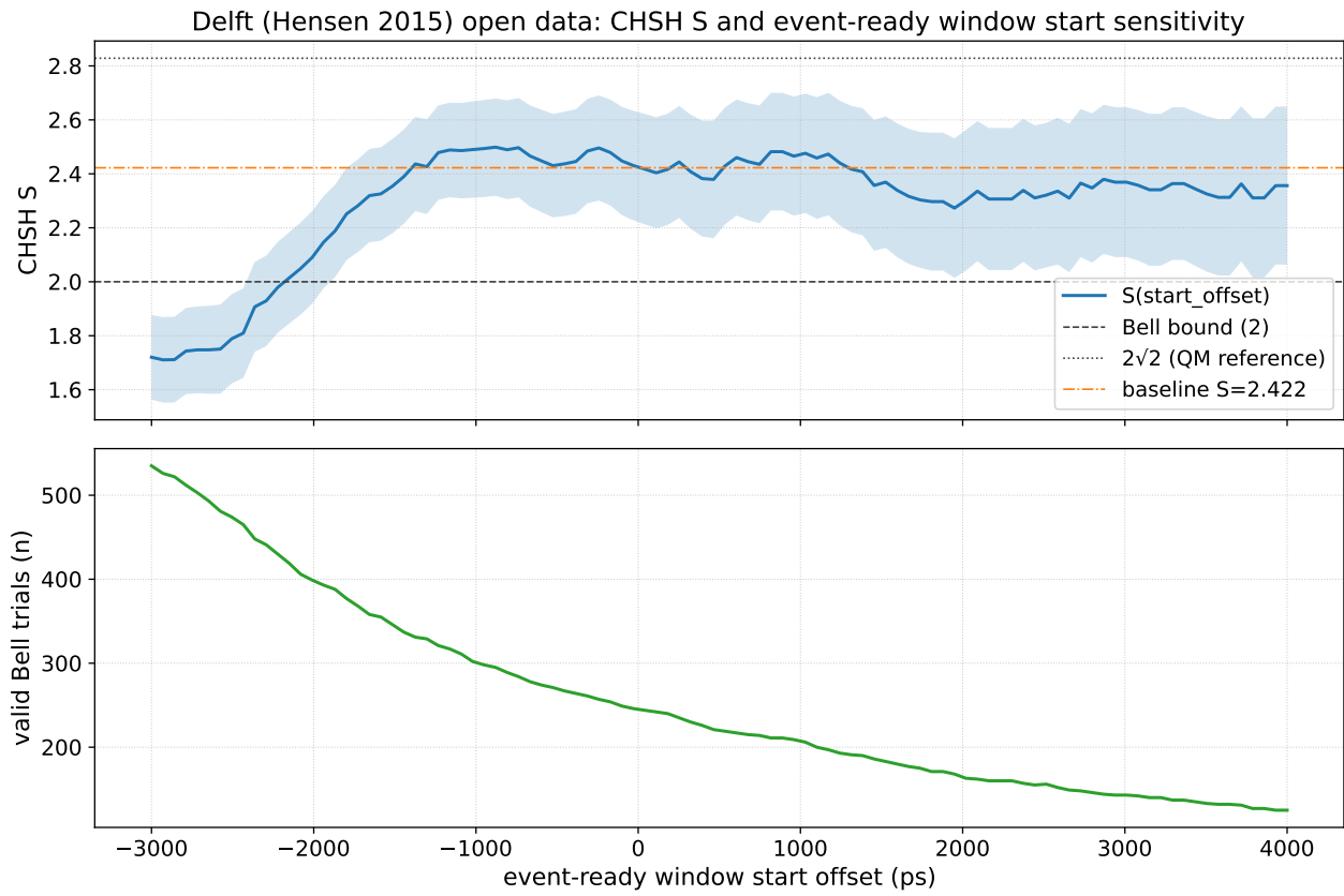
図 6: Delft 2015（事象準備型）の offset sweep に対する CHSH S の感度を示す。
