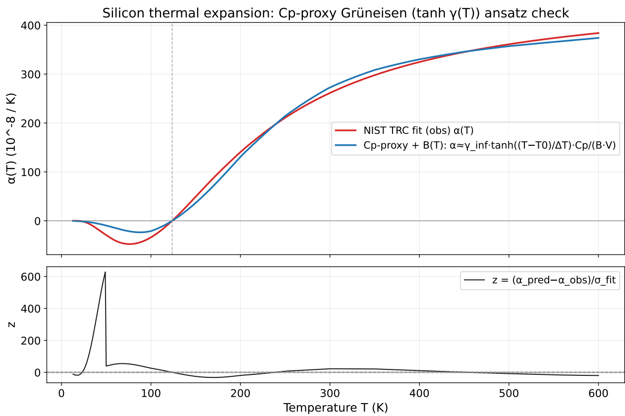
図 69: B(T) を導入しても支配的な不一致は解消しないことを示す。
