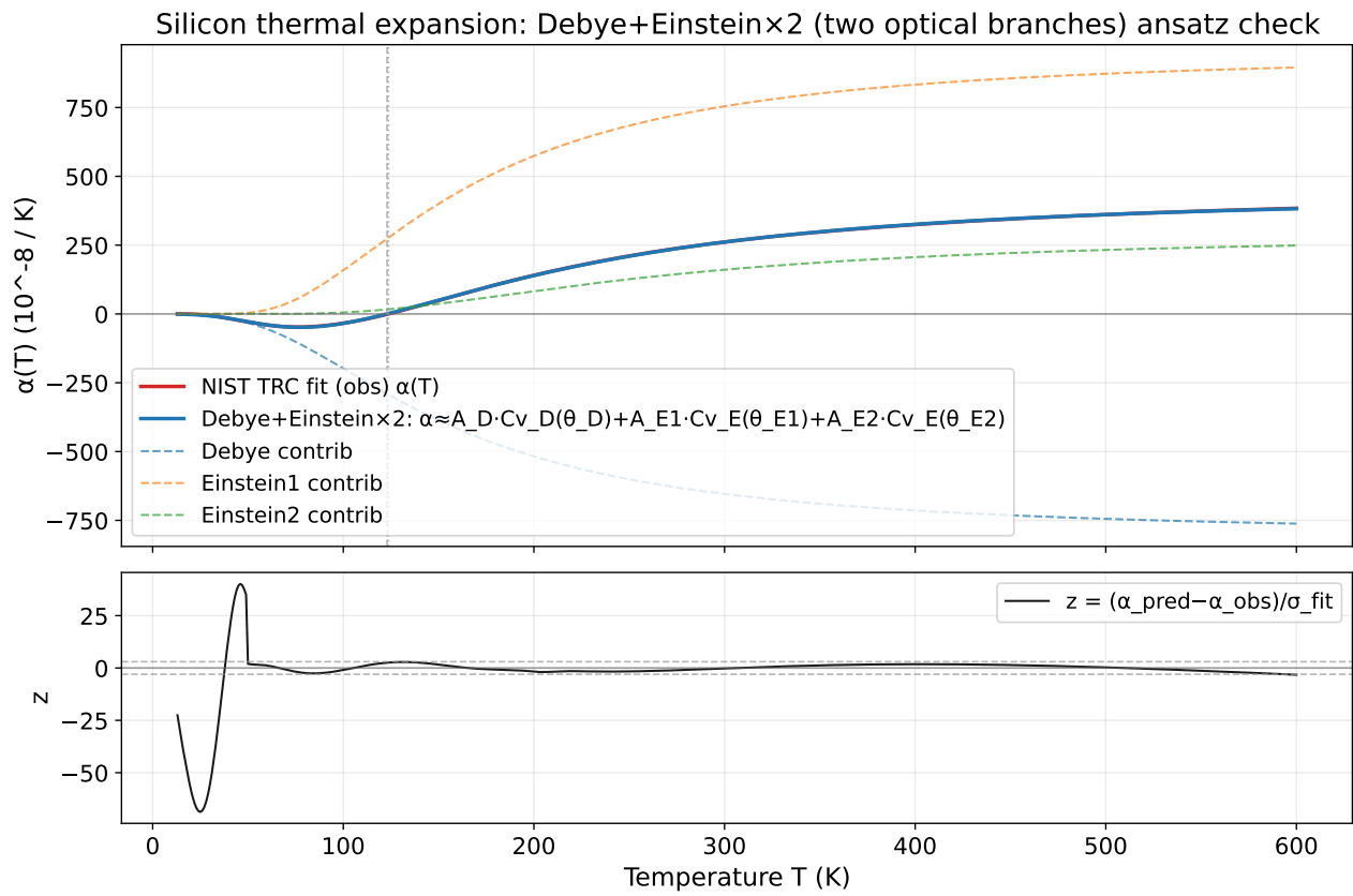
図 70: Einstein 2 枝まで増やしたときの改善量と、strict 未達を示す。
