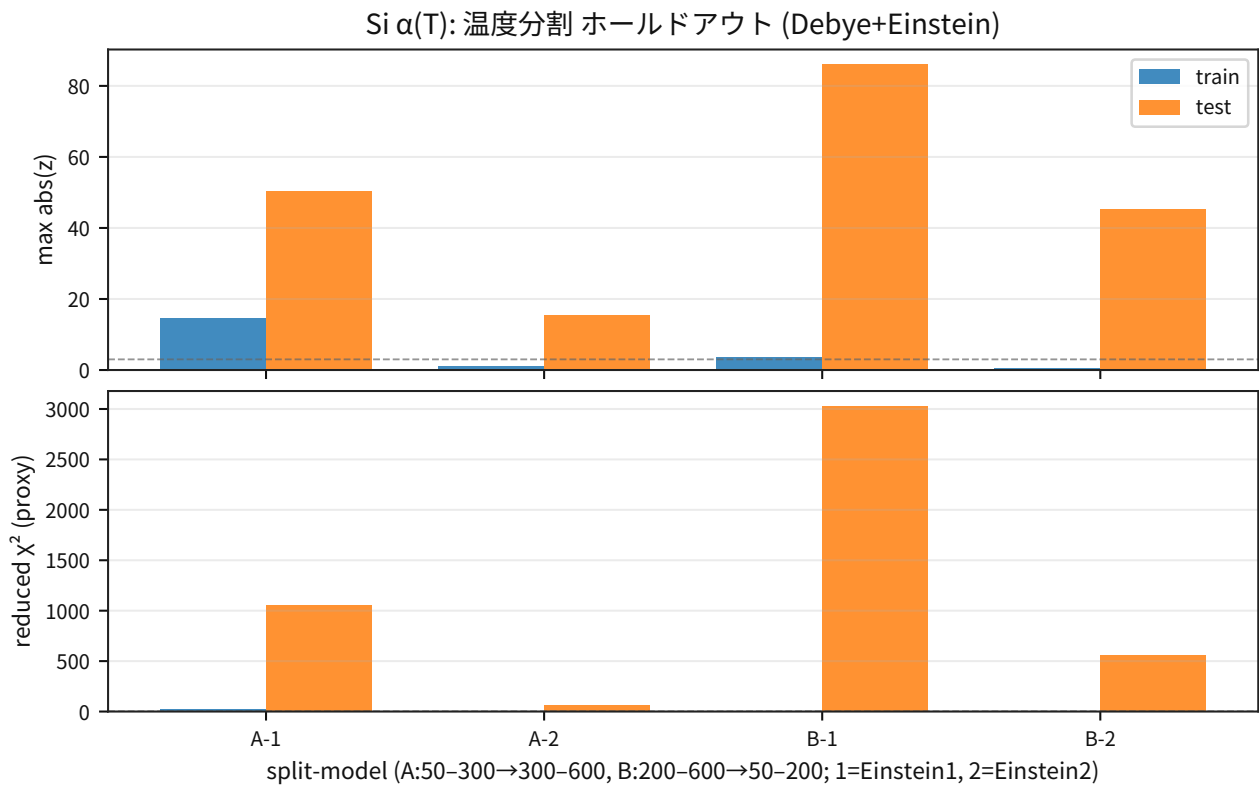
図 59: Si 熱膨張の holdout 分割監査
