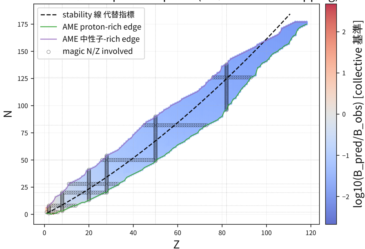
図 55: AME2020 全核種の Z-N 残差マップ
