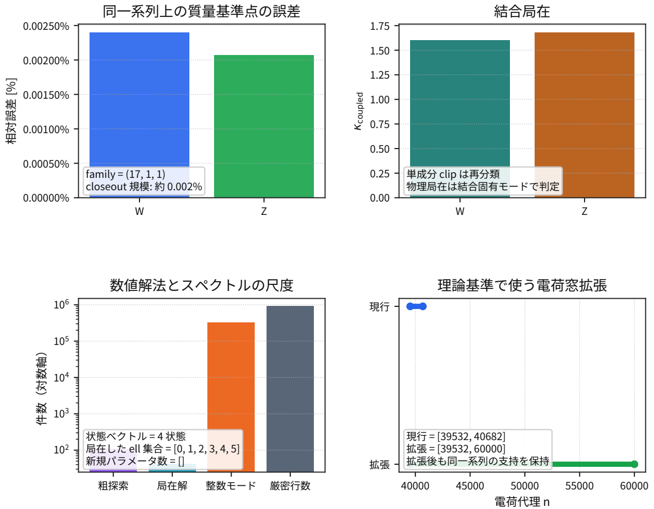
図 49: W/Z 質量基準点の結合局在条件による理論基準
