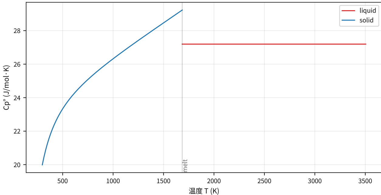
シリコン 熱容量 (Shomate; NIST WebBook condensed 位相)
