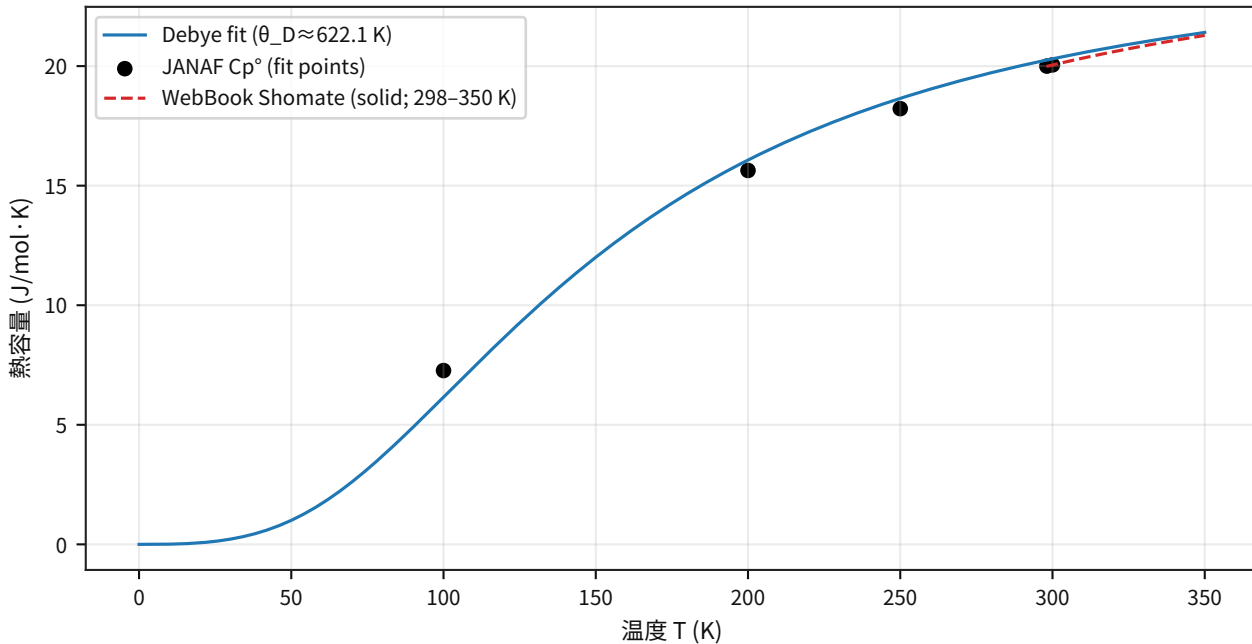
シリコン 熱容量: JANAF 基準 + Debye-fit 目標 (low T)
