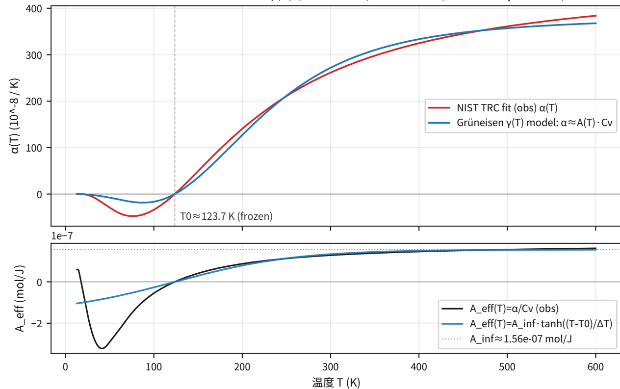
シリコン 熱膨張: minimal \gamma(T) (Grüneisen) extension (tanh interpolation)
