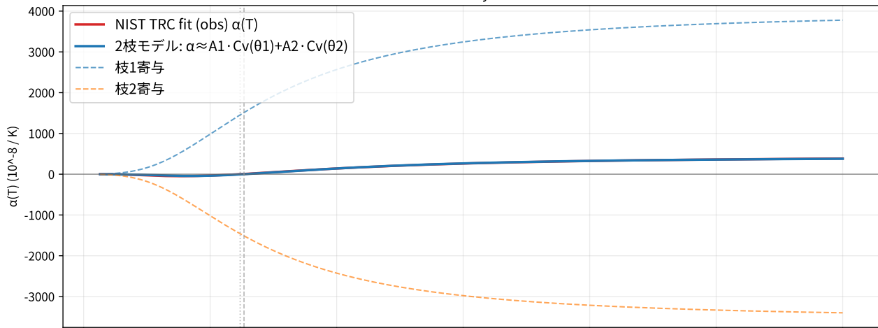
シリコン熱膨張: 2枝 Debye-Grüneisen モデル
