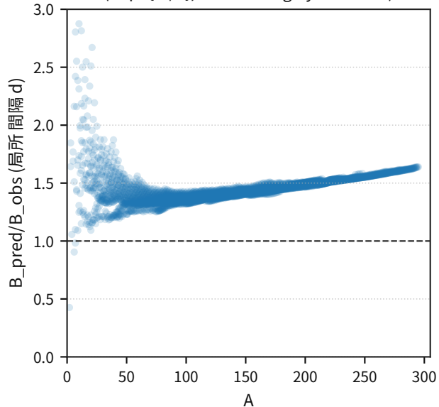
局所 間隔 代替指標 ( d=\rho^{-1/3} ; A-trend largely removed)
