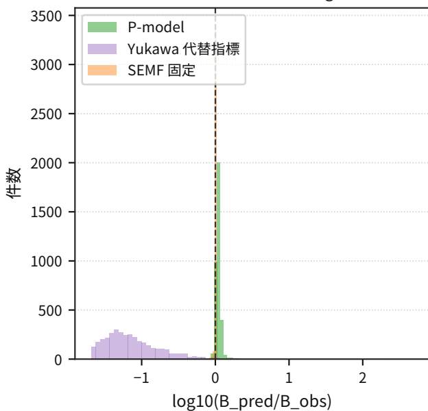
残差 distributions in common log10 スケール
