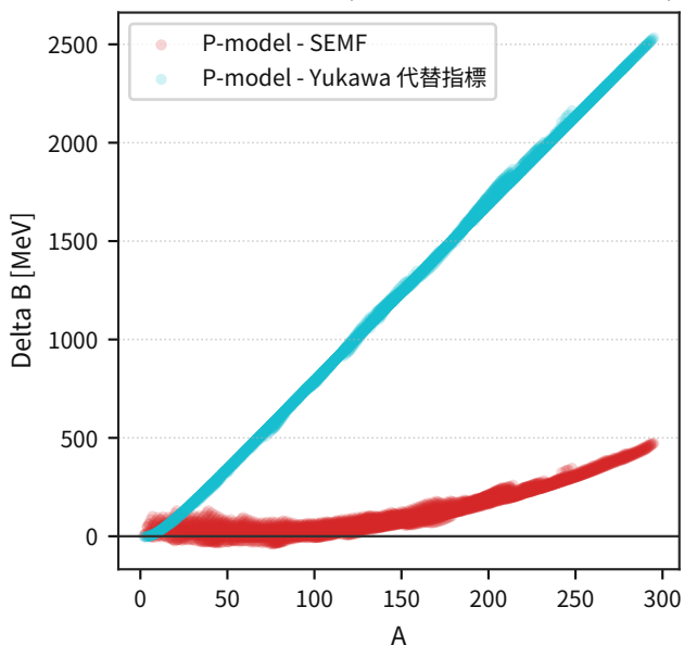
差分 予測 チャンネル (same AME2020 ターゲット)
