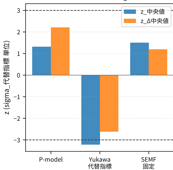
運用 整合性 下で 凍結 3sigma 閾値
