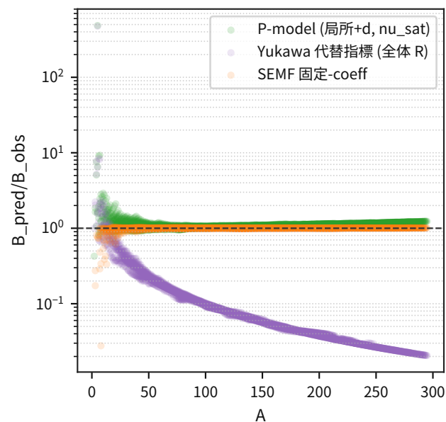
All-nuclei 残差 スケール による モデル class
