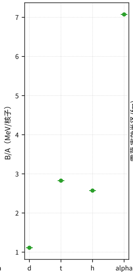
核子当たり結合エネルギー
