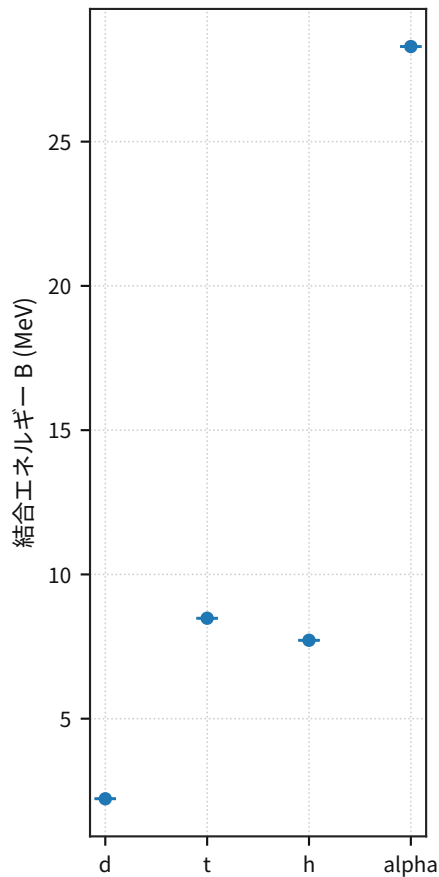
質量欠損の基準（CODATA/NIST）
