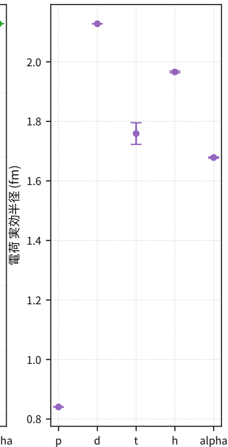
電荷半径（CODATA + IAEA 集約）
