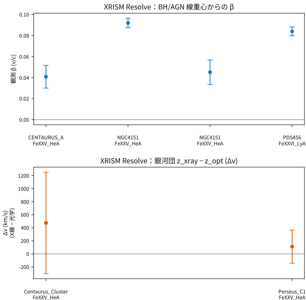
図 29: Resolve の BH/AGN ( \beta_{\text{obs}} ) と銀河団 ( \Delta v の proxy) の代表結果を俯瞰する。
