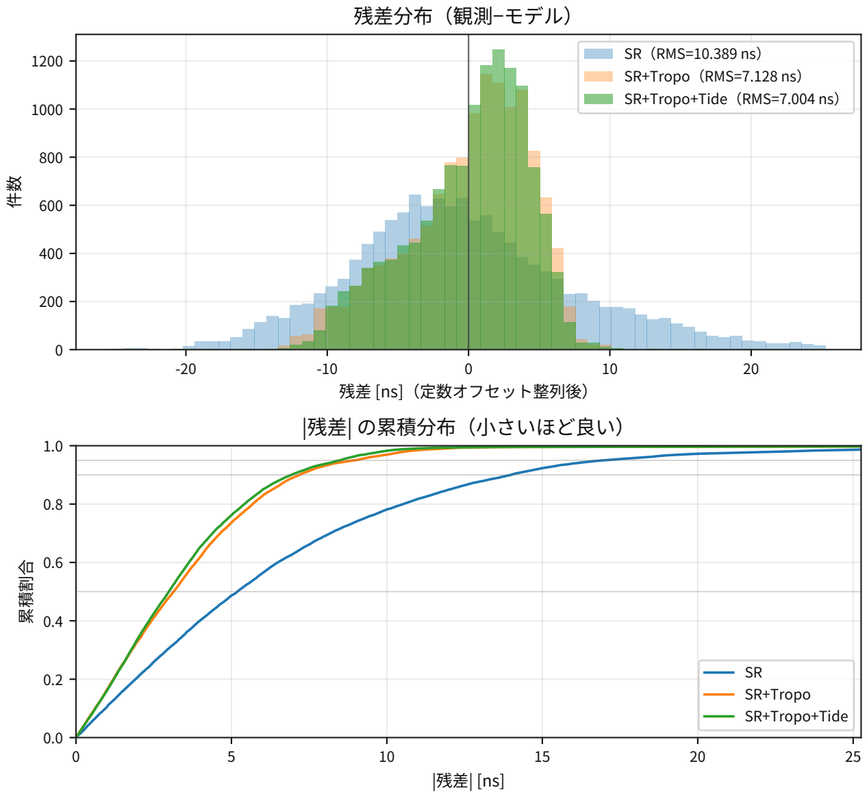
図 4: 残差分布（RMS/外れ値）を段階追加で比較し、収束と尾の変化を確認する。
