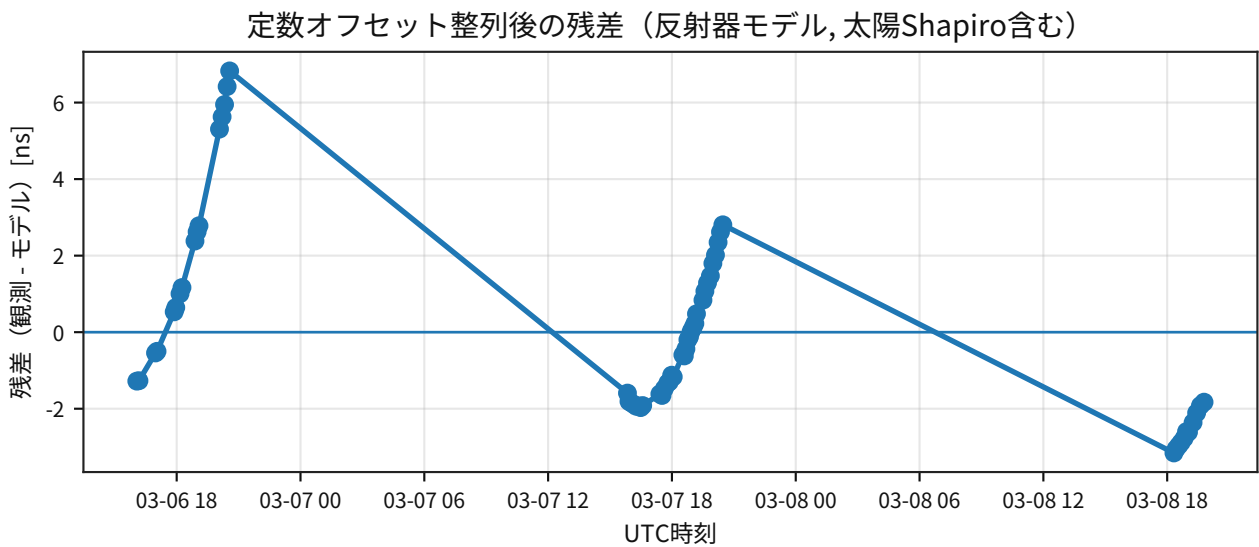
図 3: 観測－モデル残差の代表図（差分を直接可視化）。
