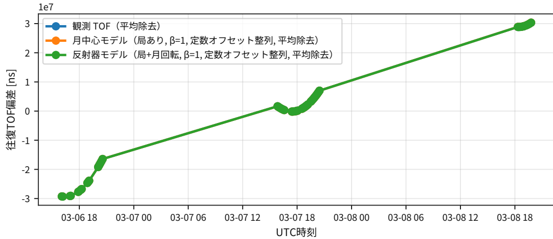
図 2: 観測 ToF とモデル ToF の重ね描き（全体のスケール整合の確認）。
