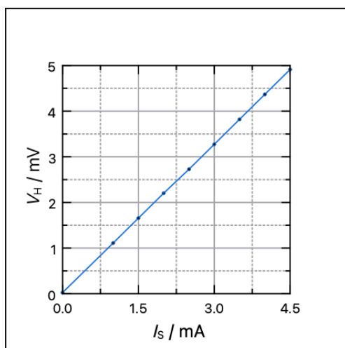
Figure 1. 固定励磁电流 I_M = 0.45 \text{ A} 不变时, 绘制得 V_H - I_S 的关系图线.
