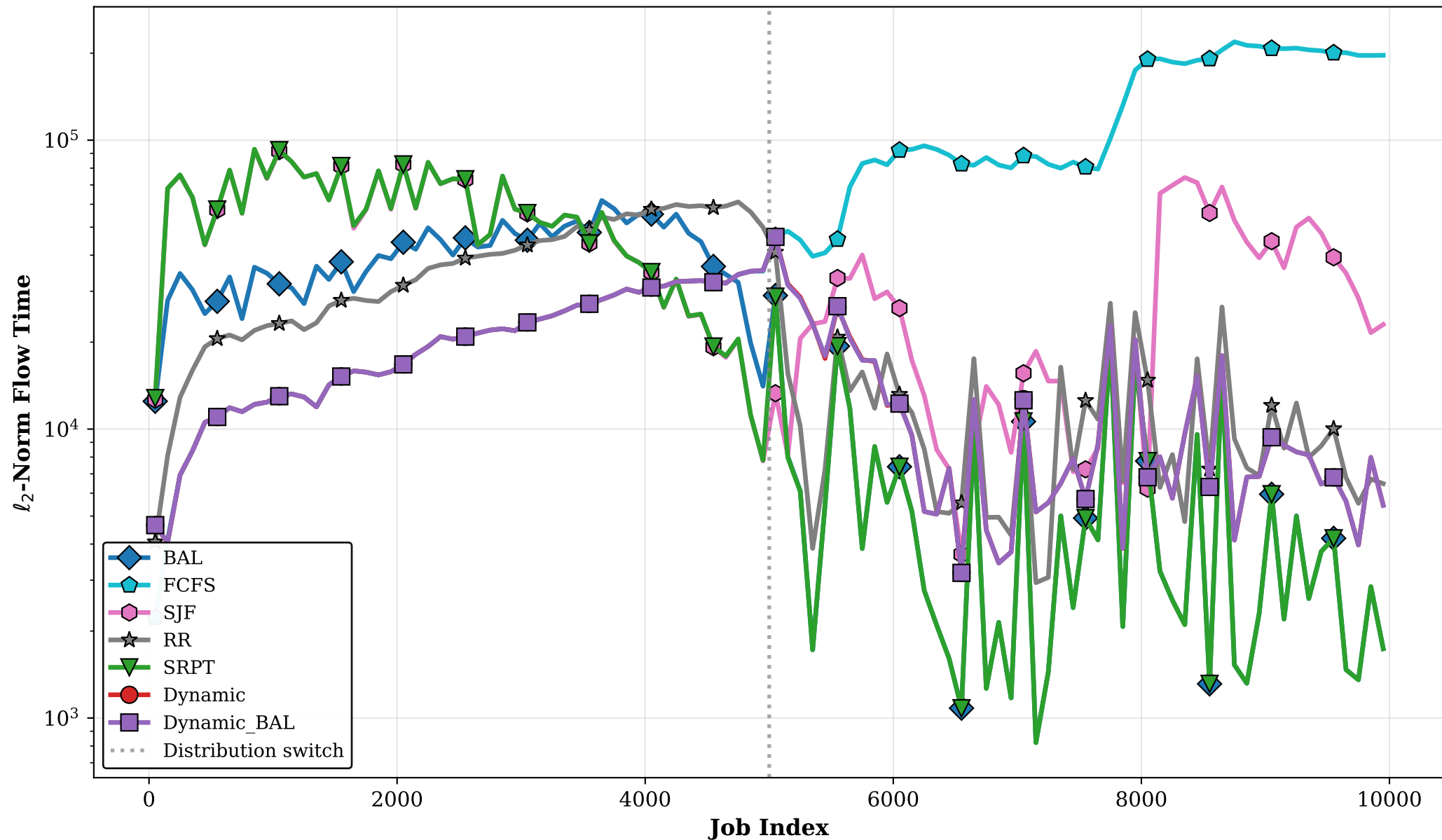
Clairvoyant Distribution Shift BP- H = 2^6 (first 5k) \rightarrow BP- H = 2^{18} (last 5k)
