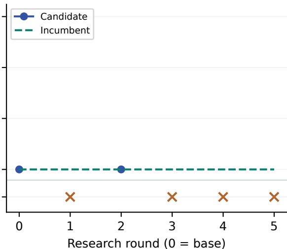
gpt-6-luna
