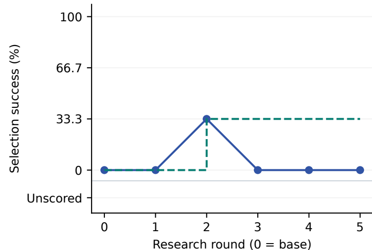
gpt-6-sol
