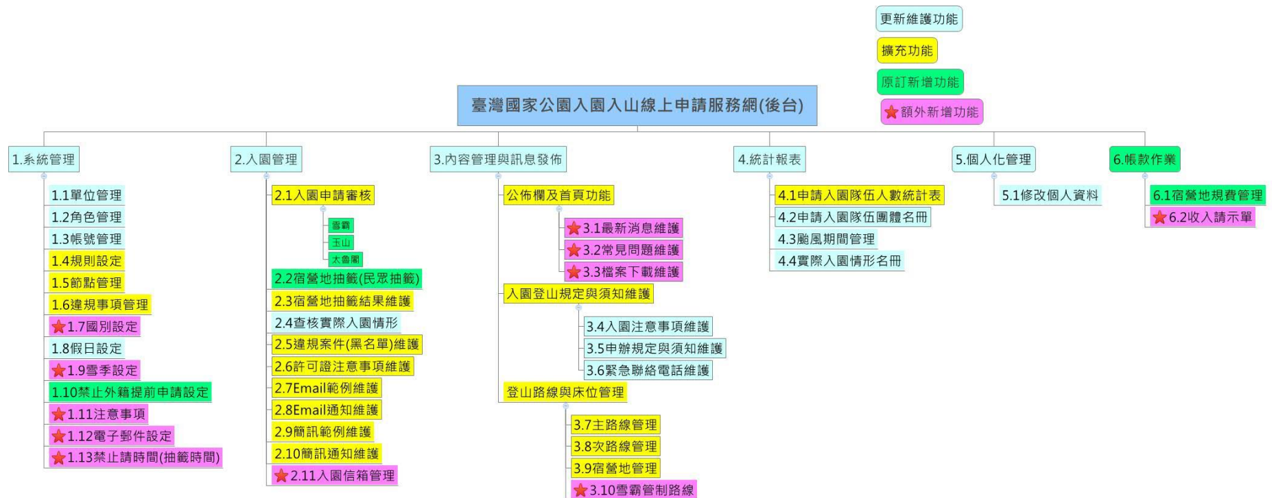
圖 1 系統功能架構圖
