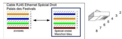
Figure 40 : Schéma d'utilisation du câble RJ45 Spécial Droit « bleu »
