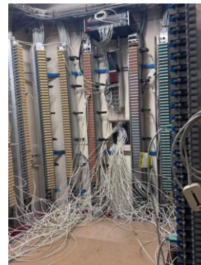
Figure 3 : Répartiteurs de l'allée 15
