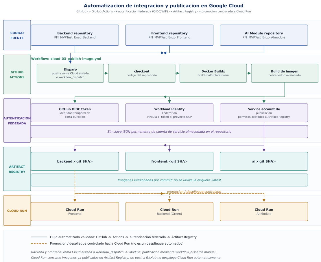
Figura 12.2: Flujo automatizado de construcción y publicación de imágenes de contenedor mediante GitHub Actions, Workload Identity Federation y Artifact Registry. La promoción hacia Cloud Run se mantiene como una acción controlada. Fuente: elaboración propia.
