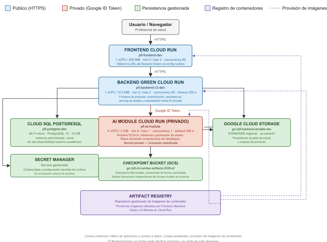
Figura 10.7: Arquitectura de despliegue validada en Google Cloud y servicios gestionados asociados. Fuente: elaboración propia.
