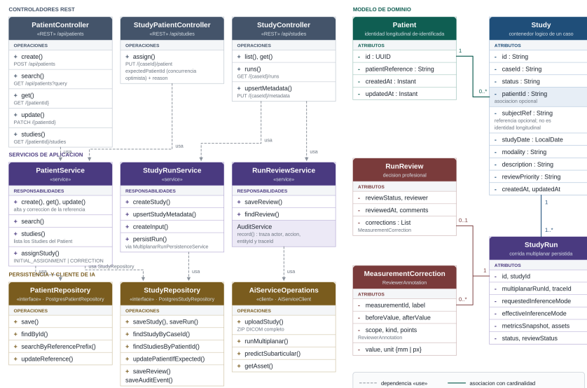
Figura 10.5: Diagrama de clases del dominio y servicios. Fuente: elaboración propia. la persistencia y reapertura, y la comunicación entre servicios.
