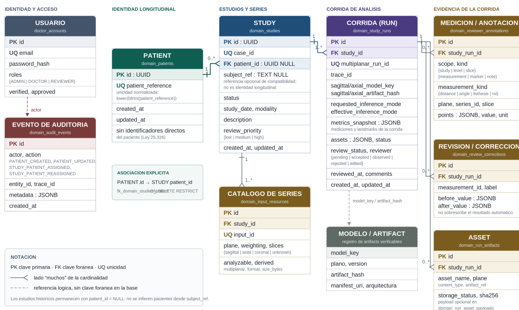
Figura 10.4: Modelo de datos relacional (PostgreSQL). Fuente: elaboración propia.
