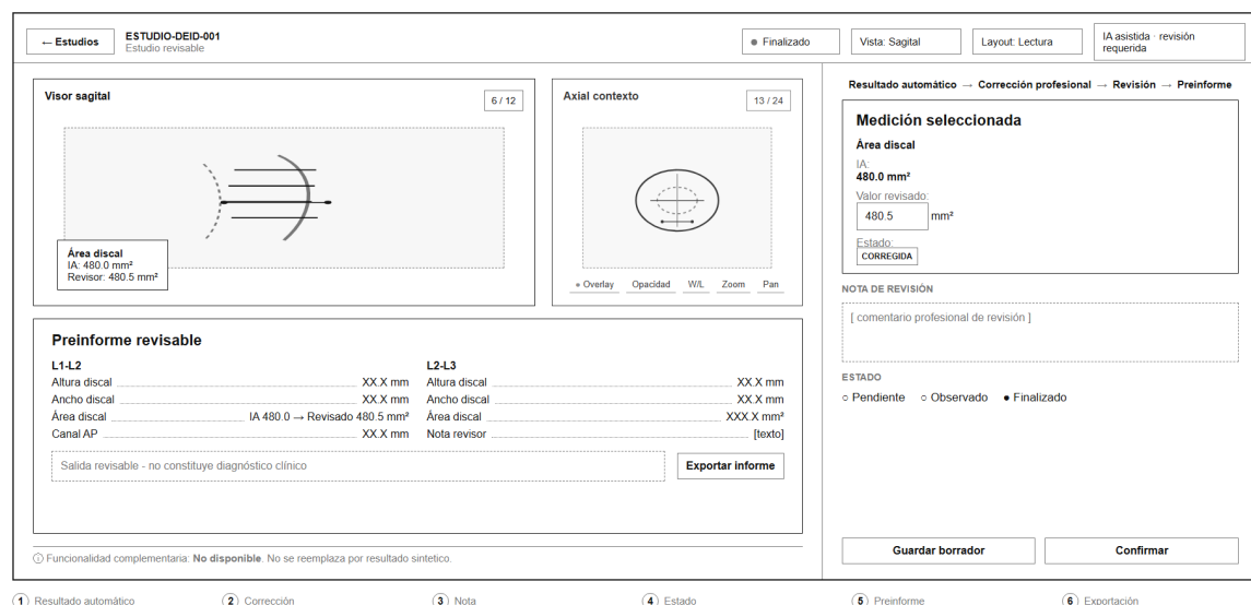
Figura 10.9: Wireframe de baja fidelidad del flujo de revisión profesional y preinforme, mostrando la trazabilidad entre el resultado automático, la corrección del profesional, el estado de revisión y la salida estructurada revisable. Fuente: elaboración propia.
