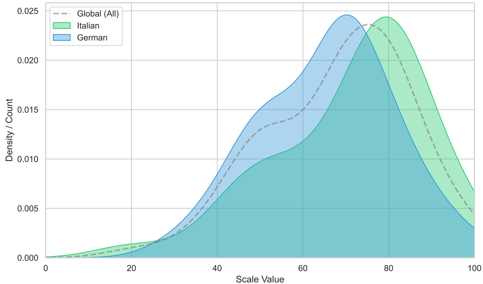
Distribution Comparison: Robot Trust Q13
