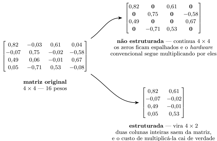
Figura 4 – As duas categorias de poda aplicadas à mesma matriz de pesos. Na poda não estruturada os pesos removidos são apenas zerados e a matriz conserva suas dimensões; na poda estruturada, colunas inteiras são eliminadas e a matriz encolhe de fato.
