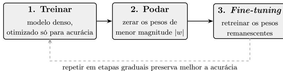
Figura 5 – Pipeline clássico de poda por magnitude: treinamento do modelo denso, remoção dos pesos de menor magnitude e retreinamento ( fine-tuning ) dos pesos remanescentes.
