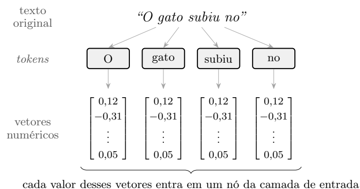
Figura 2 – Da frase aos nós da camada de entrada: o texto é fragmentado em tokens e cada token é convertido em um vetor numérico.
