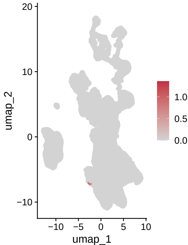
ENSG00000261080.RUNX2-AS1
