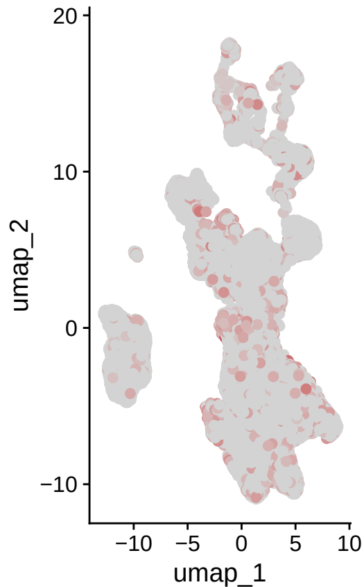
ENSG00000124813.RUNX2
