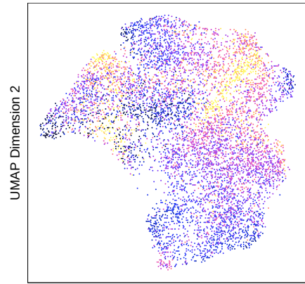
UMAP Dimension 1
