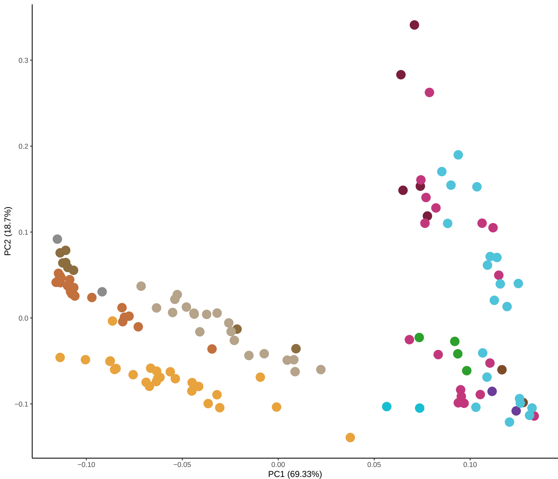
PCA mTFR_jaspar2020_distal
