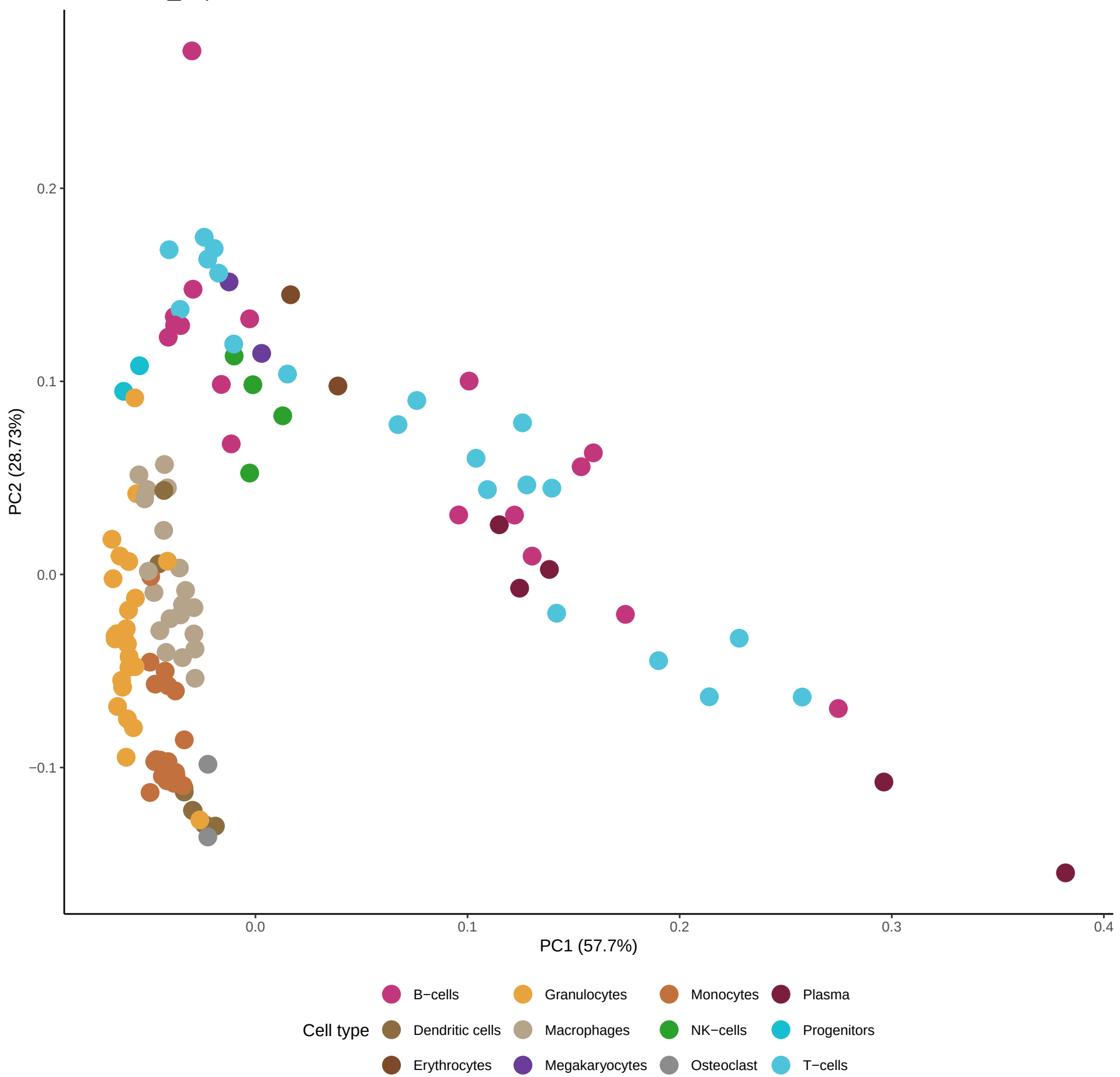
PCA mTFR_jaspar2020
