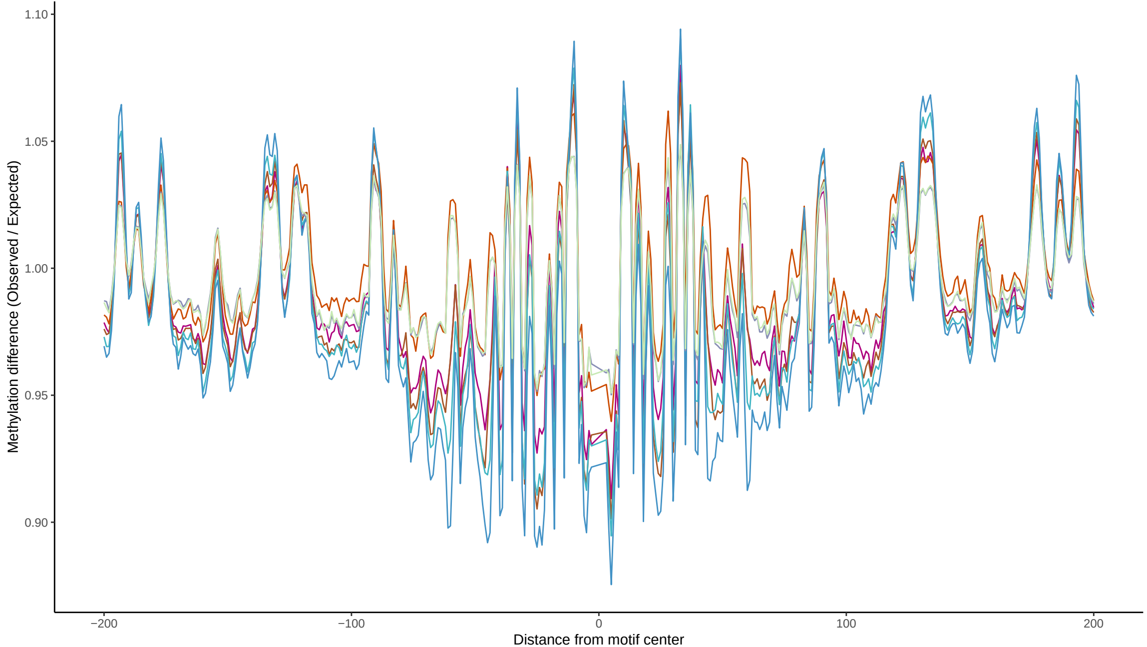
TF footprint difference for MGA
