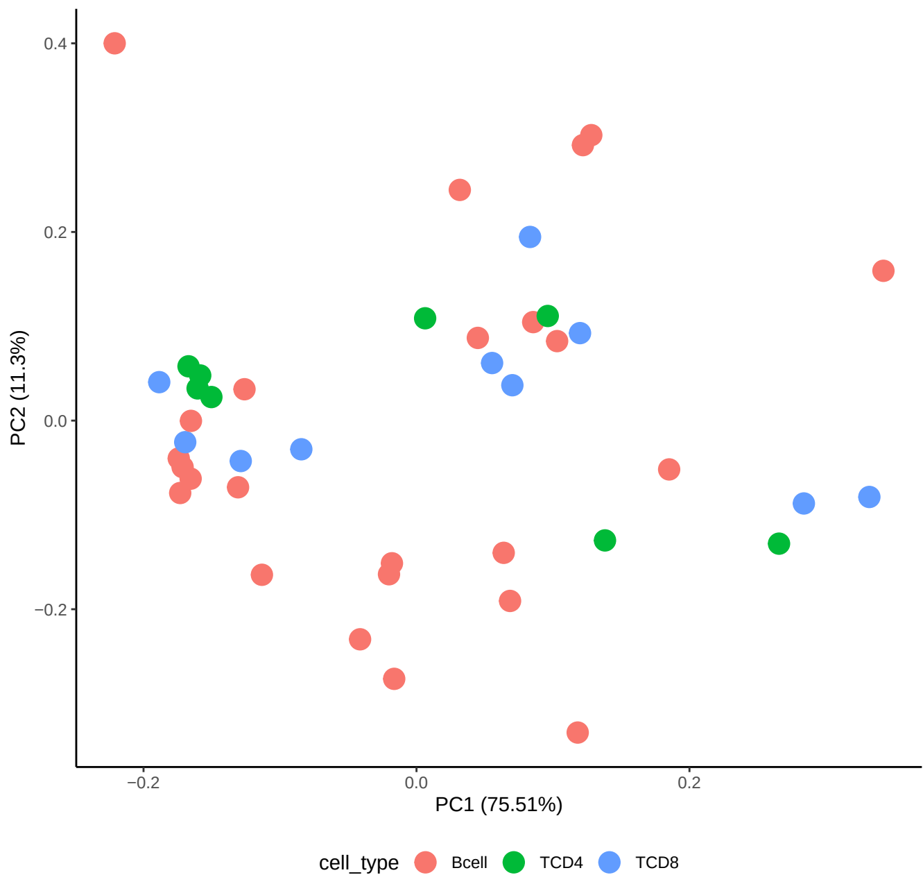
PCA – Bcell vs Tcell
