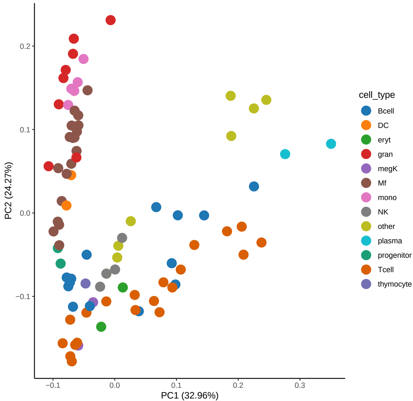
PCA – Blueprint
