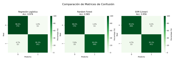
Fig. 2. Matrices de confusión para los tres modelos evaluados.
