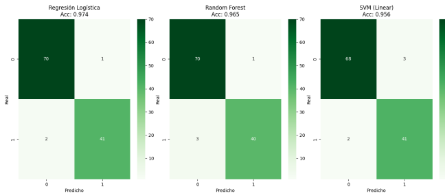
Fig. 2. Matrices de confusión para los tres modelos evaluados.
