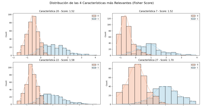
Fig. 1. Histogramas de las características más relevantes según Fisher Score.
