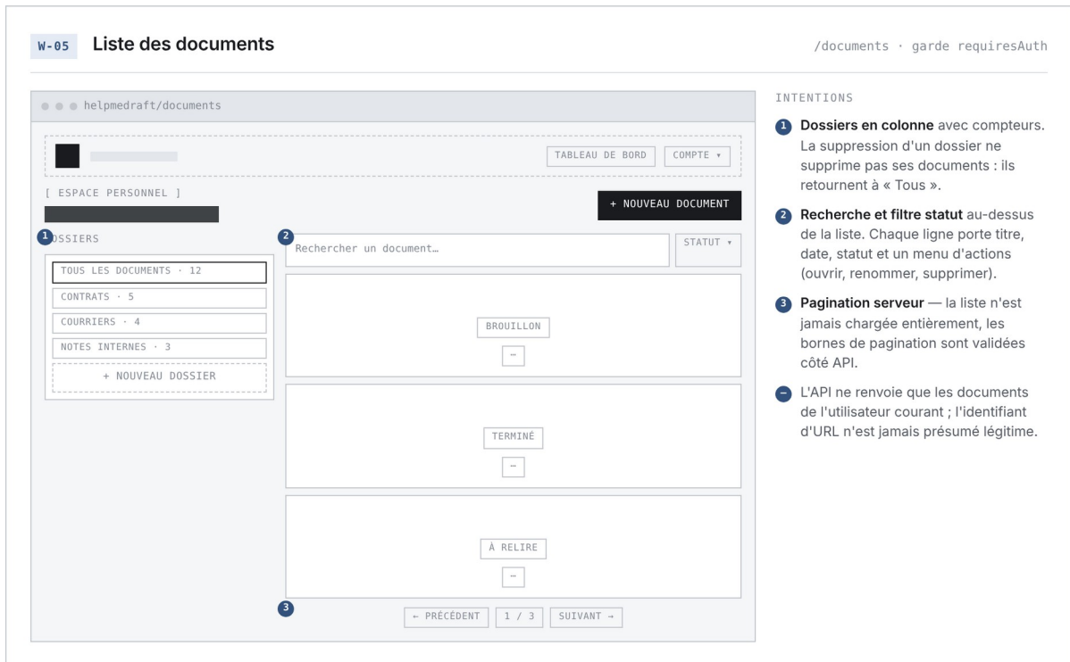
W-05 — Liste des documents (/documents). Colonne dossiers, recherche et filtre statut, pagination serveur.
