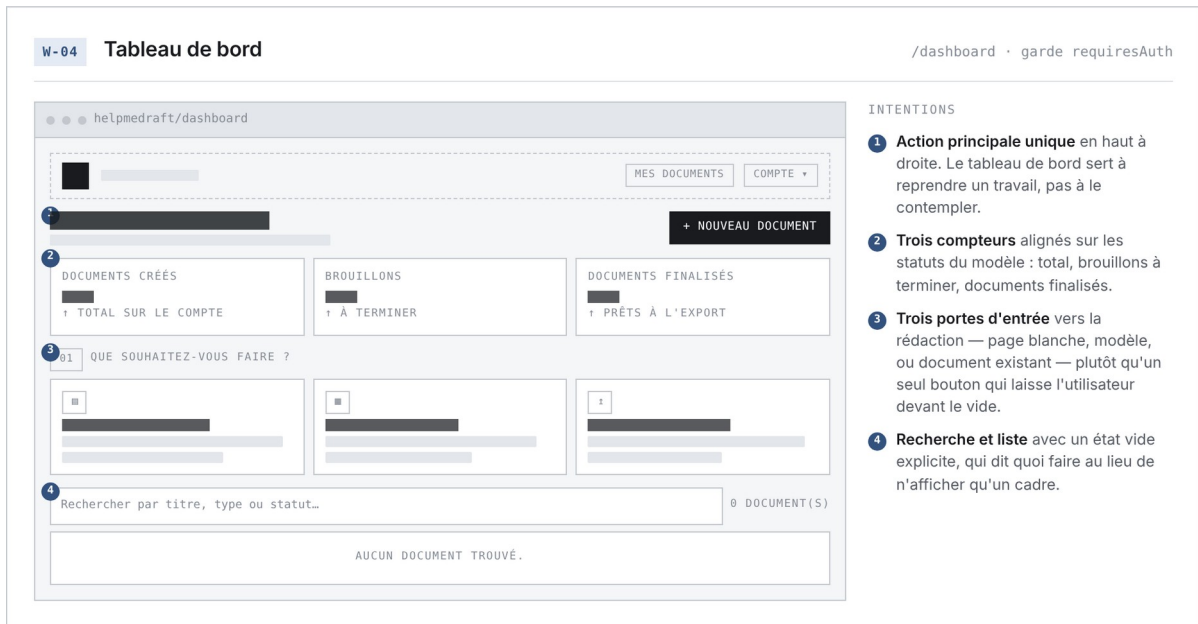
W-04 — Tableau de bord (/dashboard). Trois compteurs de statut, trois portes d'entrée vers la rédaction, état vide explicite.
