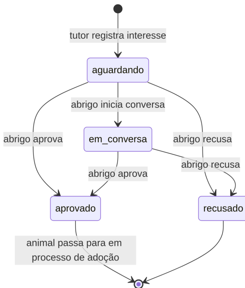
Figura 1 — Situações de um interesse de adoção e as transições permitidas
