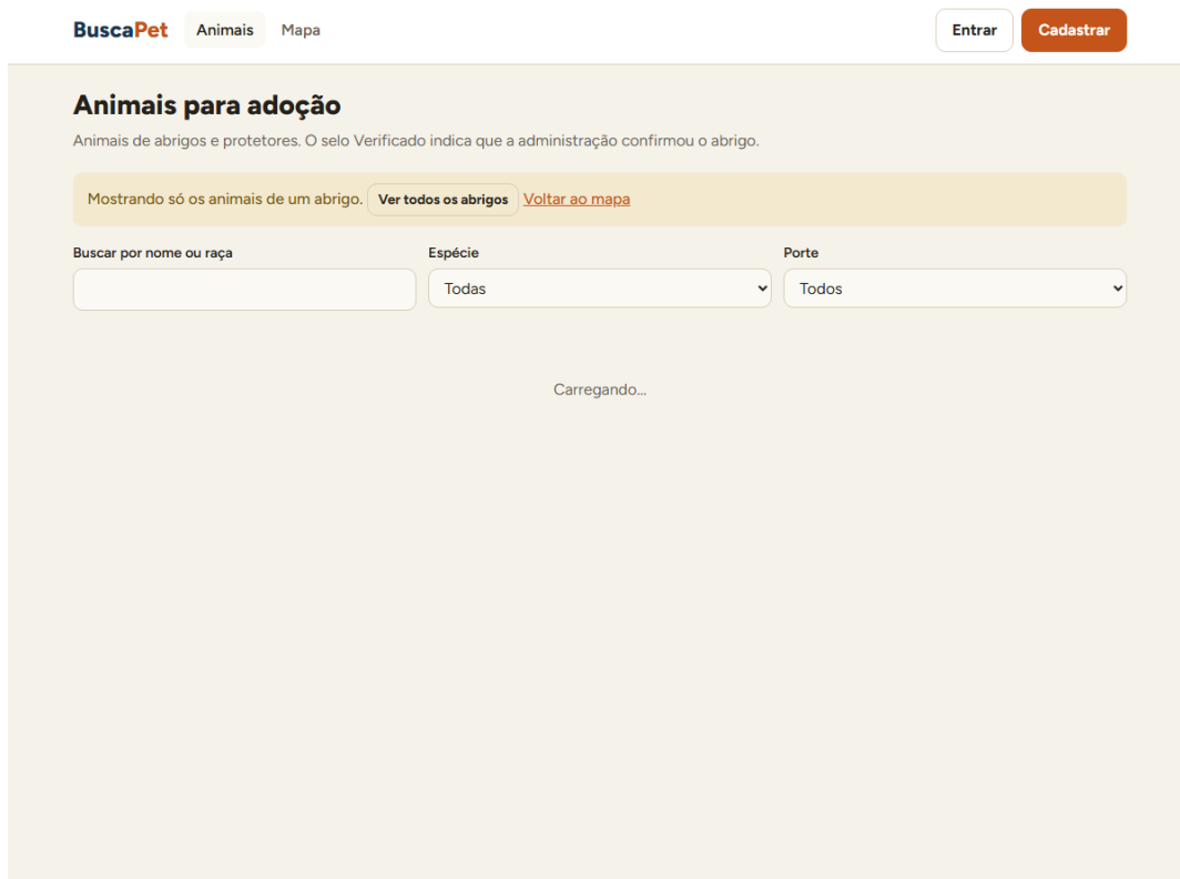
Figura 17 — “Ver animais” leva ao catálogo filtrado pelo abrigo escolhido
