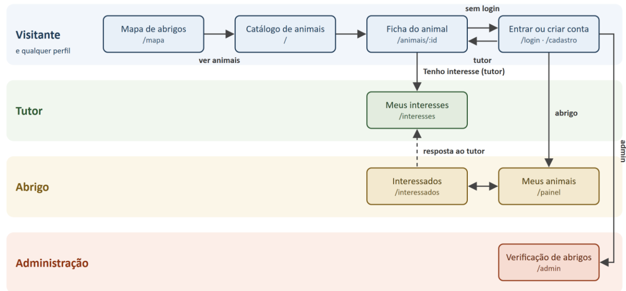
Figura 23 — Navegação entre as telas, por perfil
