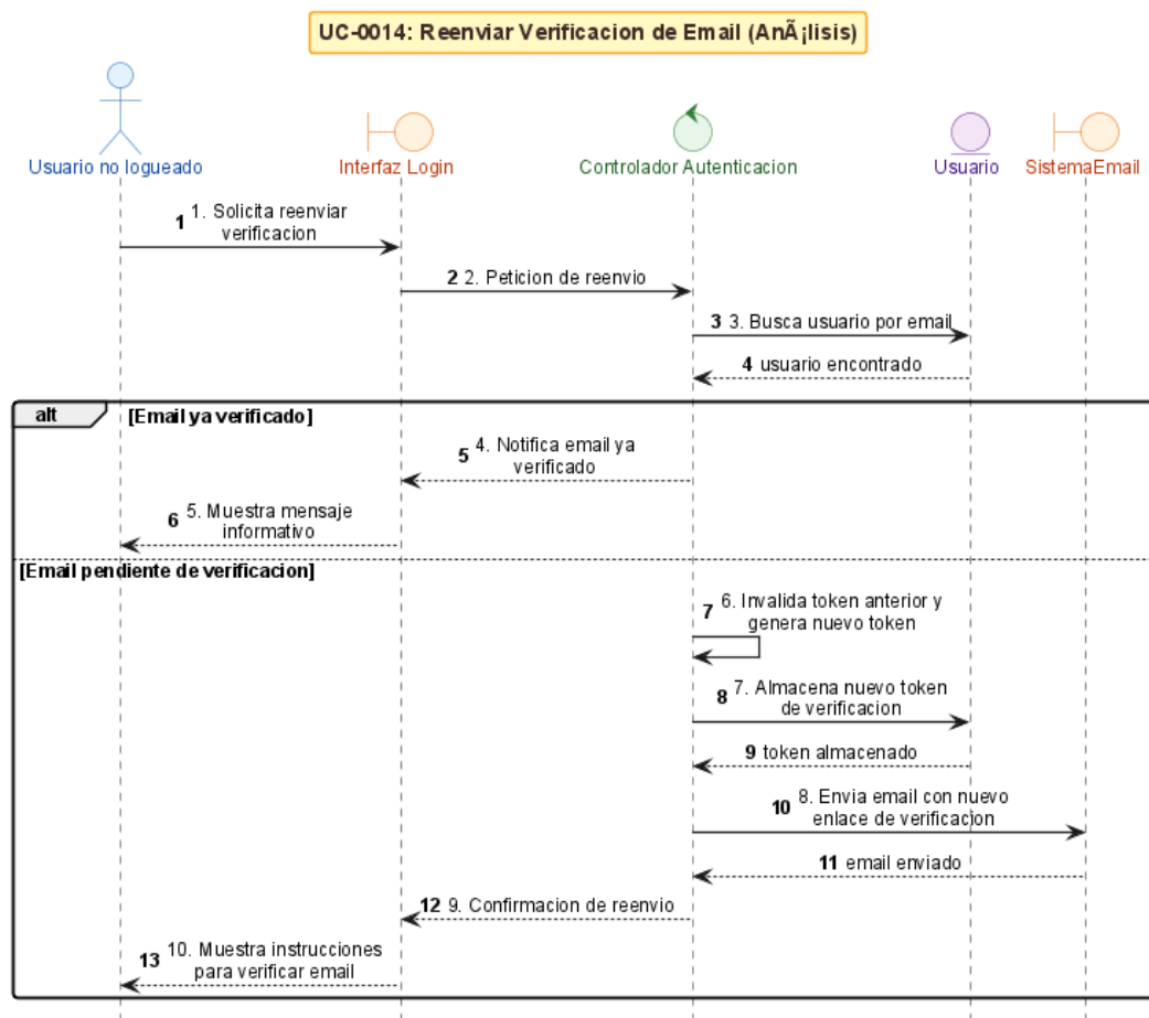
Figura 9: Diagrama de secuencia de análisis BCE – UC-0014: Reenviar Verificacion de Email
