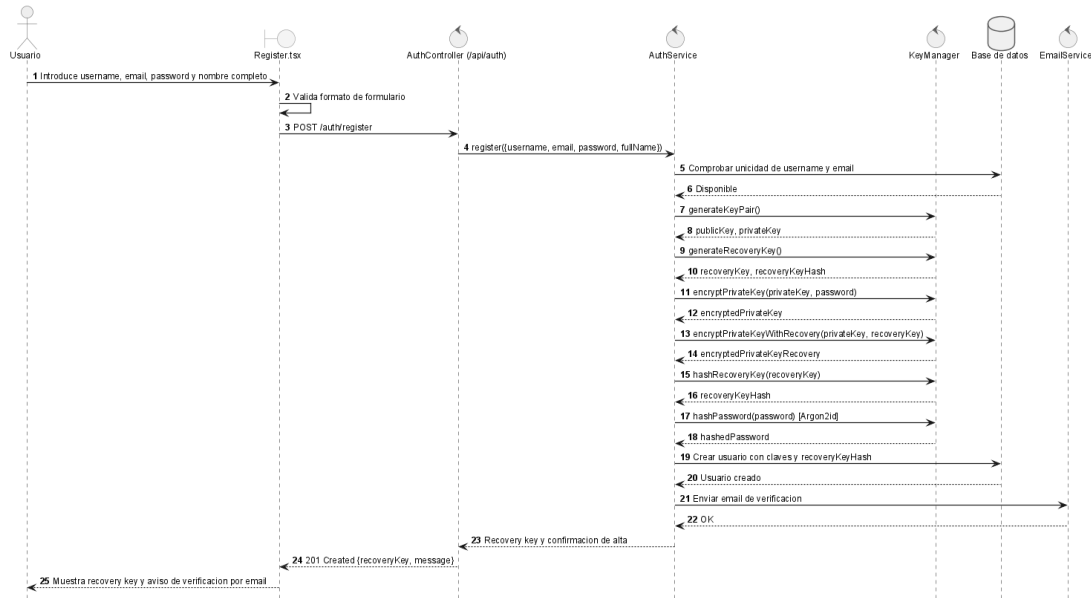
Figura 52: Secuencia de diseño — UC-0001: Registrar Usuario
