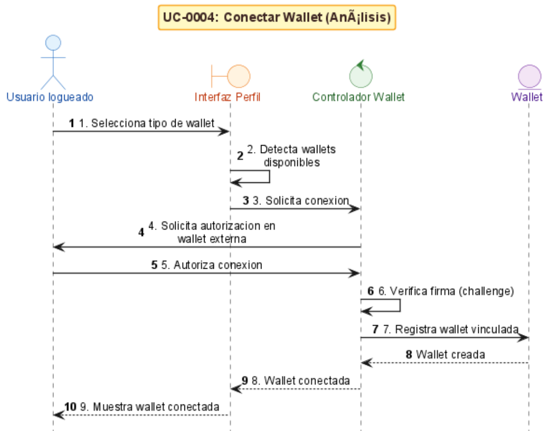
Figura 6: Análisis BCE — UC-0004: Conectar Wallet
