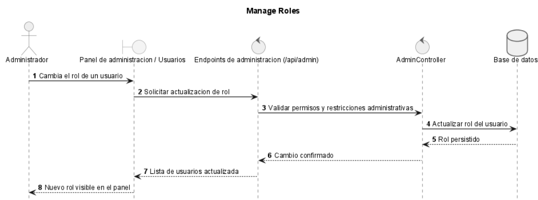
Figura 97: Secuencia de diseño — UC-0043: Gestionar Roles
