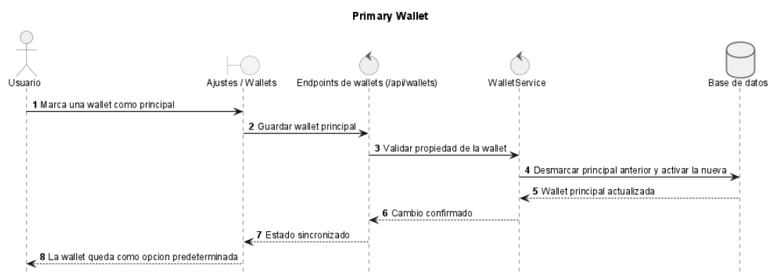
Figura 65: Secuencia de diseño — UC-0006: Wallet Principal
