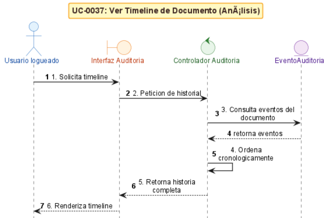
Figura 39: Análisis BCE — UC-0037: Timeline del Documento
