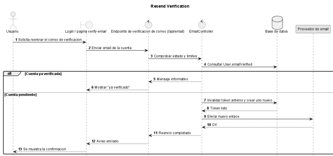
Figura 56: Secuencia de diseño — UC-0014: Reenviar Verificación
