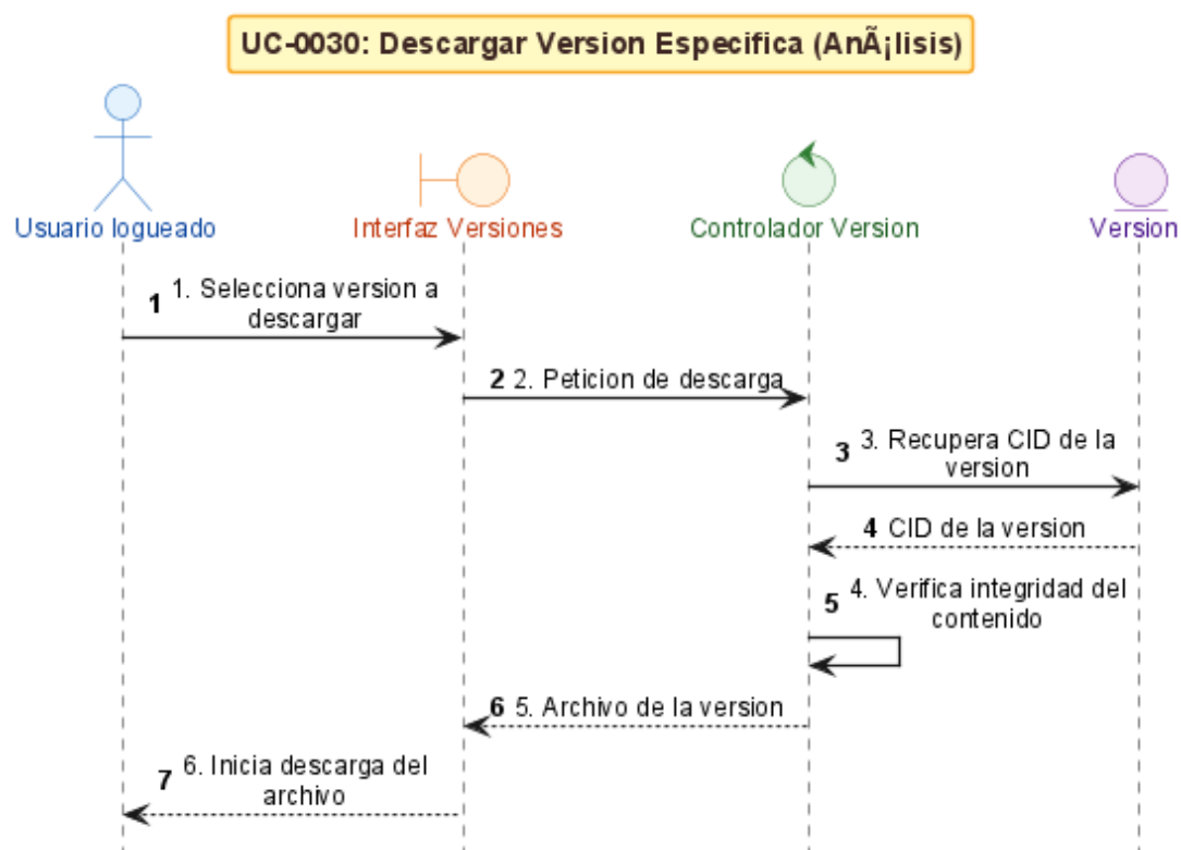
Figura 32: Análisis BCE — UC-0030: Descargar Versión
