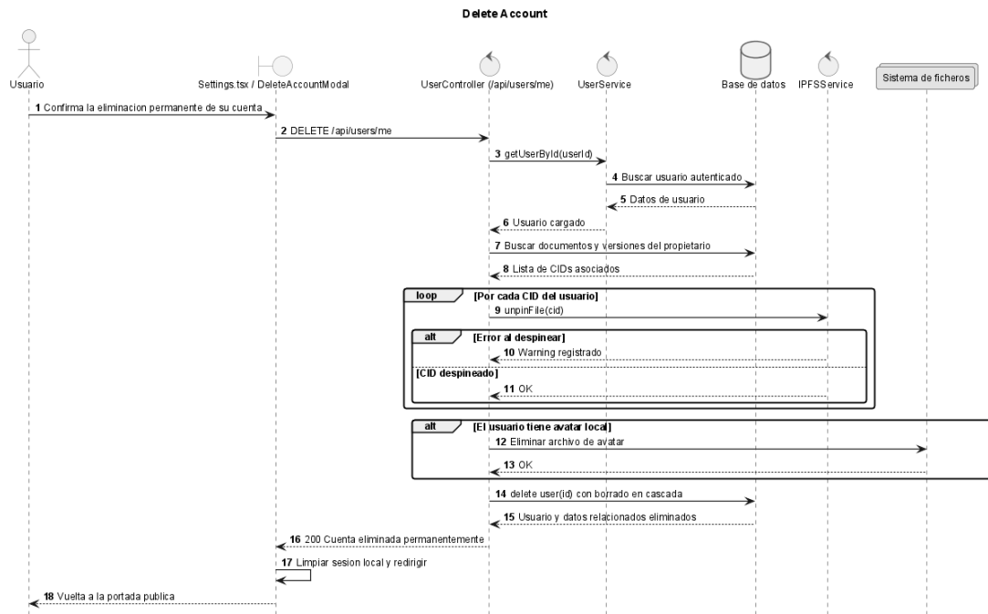
Figura 61: Secuencia de diseño — UC-0010: Eliminar Cuenta
