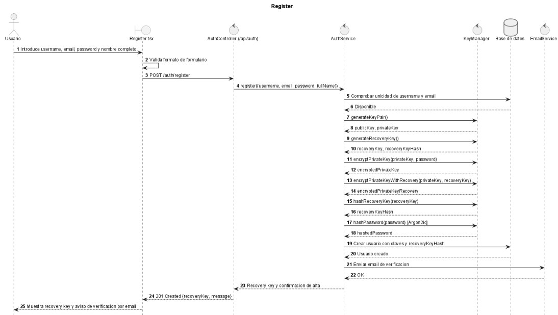
Figura 52: Secuencia de diseño — UC-0001: Registrar Usuario
