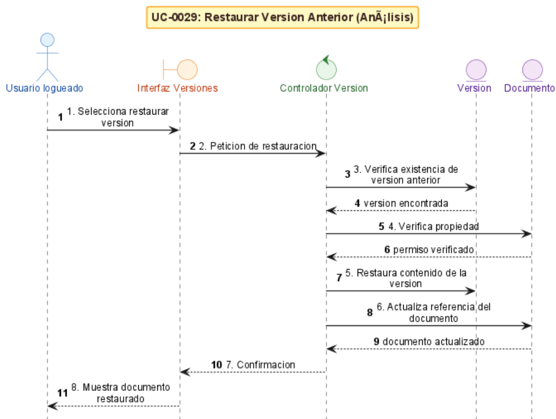
Figura 31: Análisis BCE — UC-0029: Restaurar Versión
