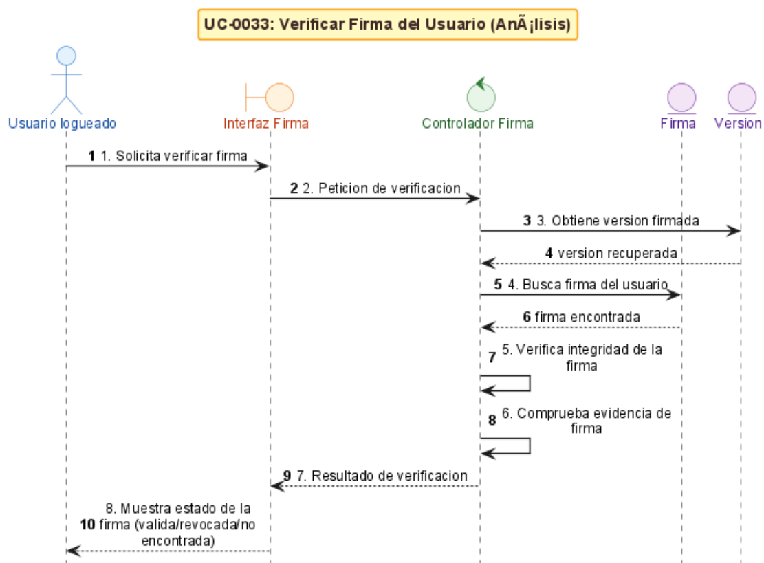
Figura 35: Análisis BCE — UC-0033: Verificar Firma
