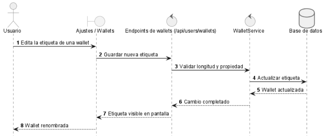
Figura 66: Secuencia de diseño — UC-0007: Renombrar Wallet
