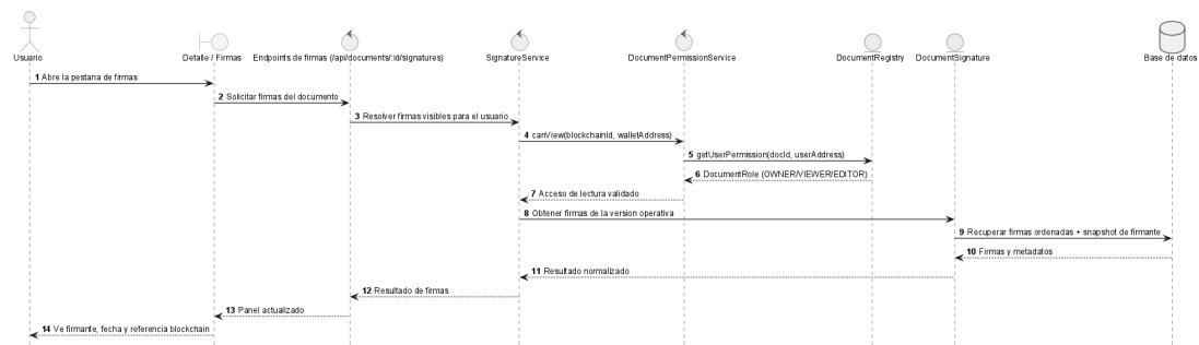
Figura 86: Secuencia de diseño — UC-0032: Ver Firmas
