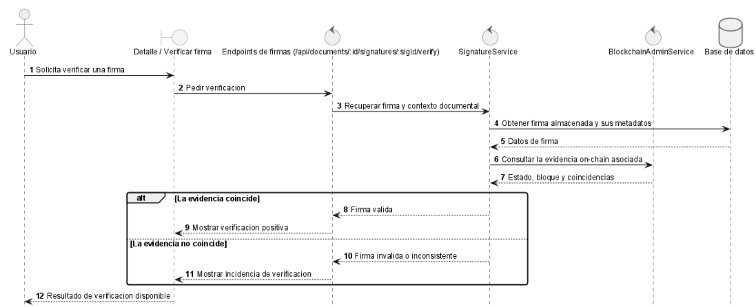
Figura 87: Secuencia de diseño — UC-0033: Verificar Firma
