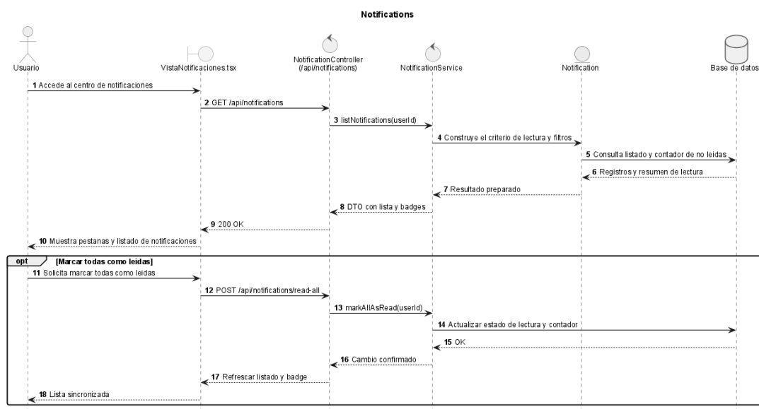
Figura 62: Secuencia de diseño — UC-0009: Consultar Notificaciones
