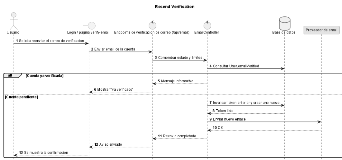
Figura 10: Diagrama de secuencia de diseno – UC-0014: Reenviar Verificacion de Email
