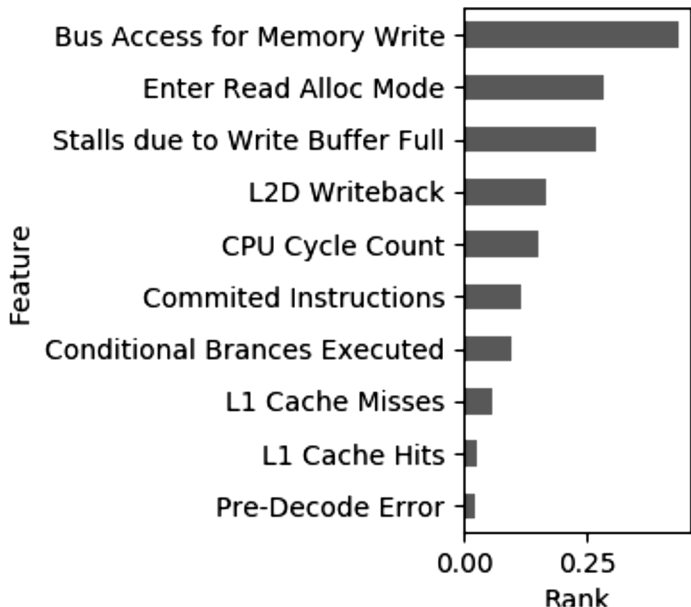
Lasso CV Feature Rank
