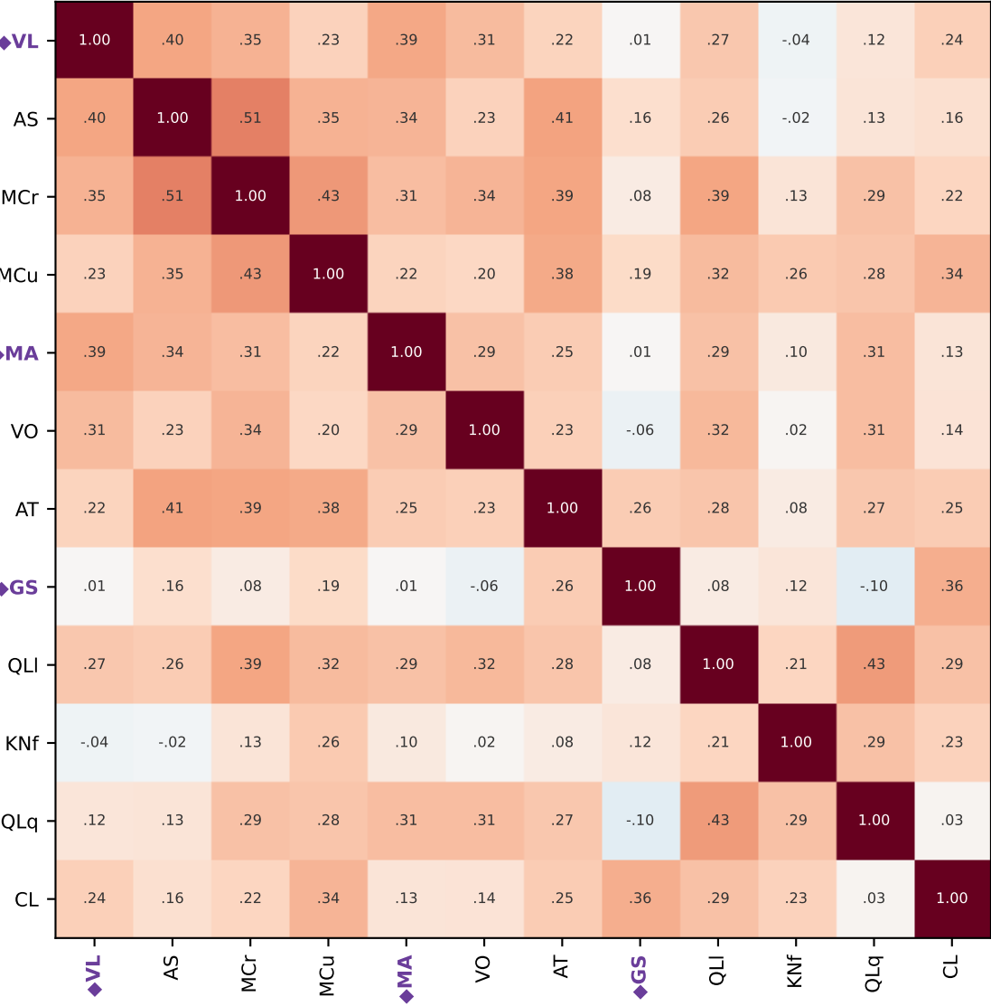
CORRECT (n=237)
