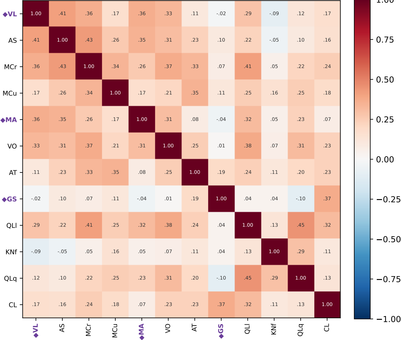
INCORRECT (n=549)
