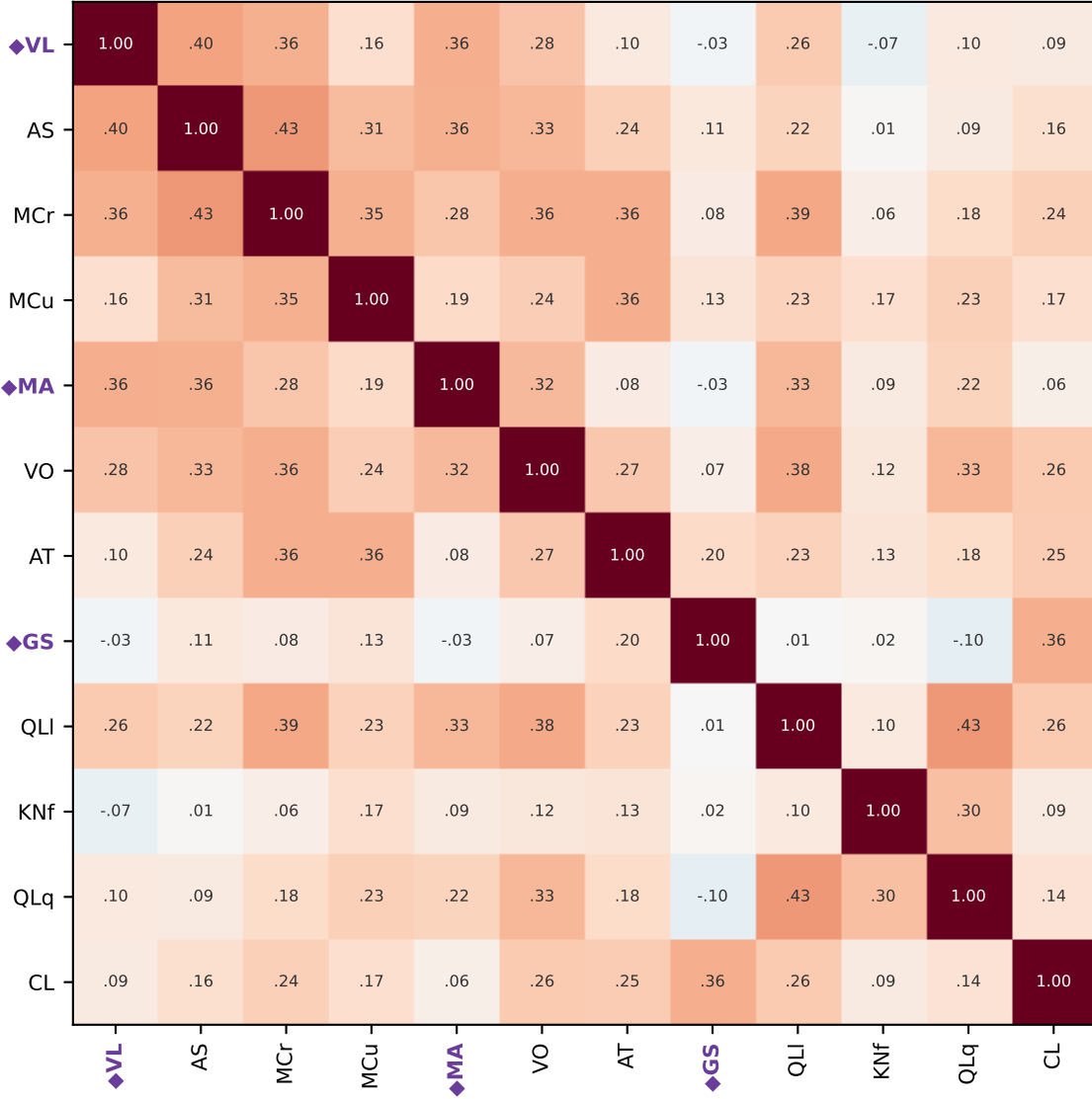
INCORRECT (n=562)
