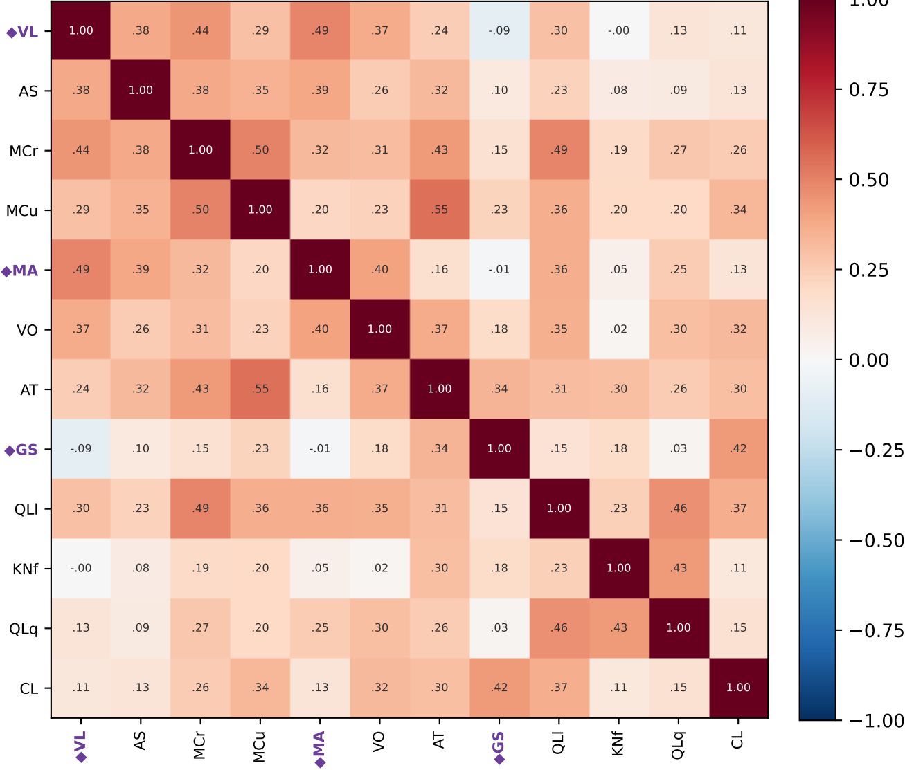
INCORRECT (n=154)
