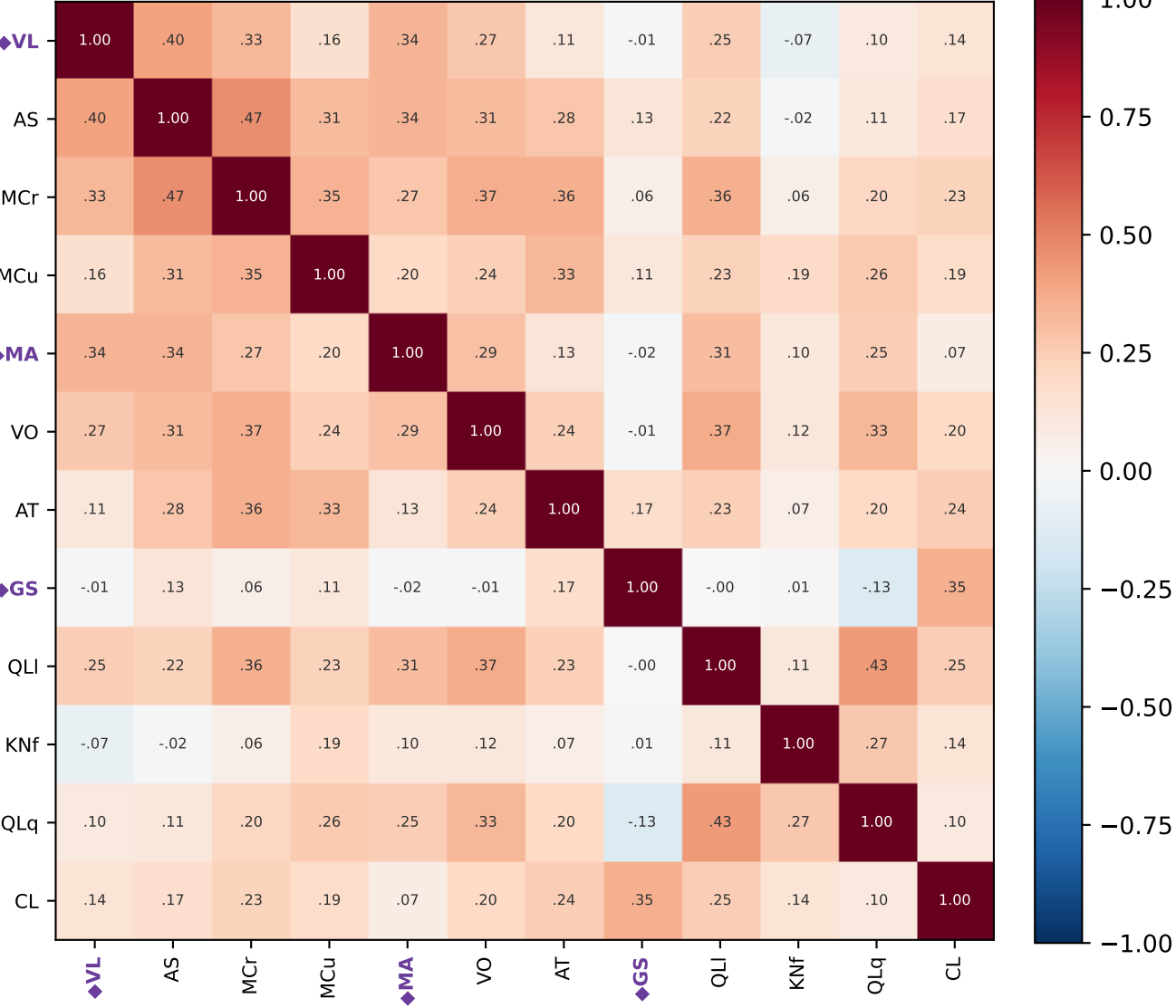
CORRECT (n=646)
