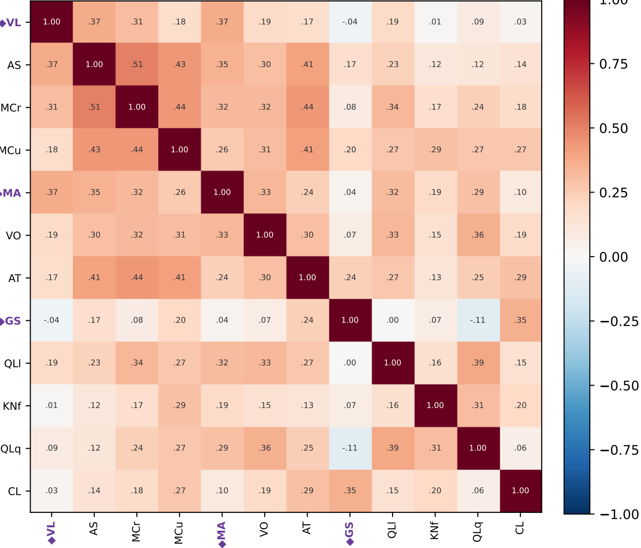
CORRECT (n=251)
