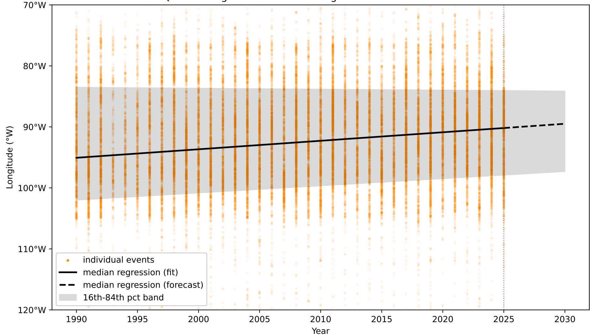
Quantile Regression: Tornado Longitude Trend & 2030 Forecast
