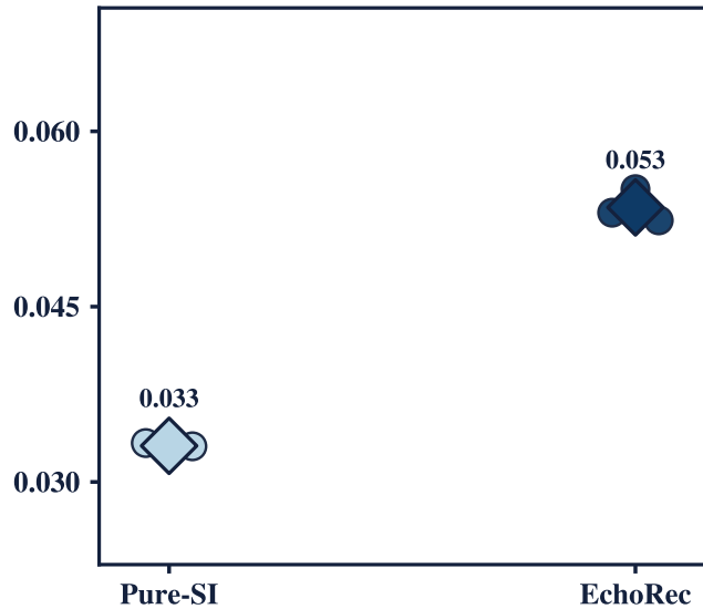
SRec-Semantic Jaccard@20
