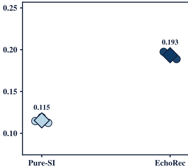
SRec-to-LLM Jaccard@20
