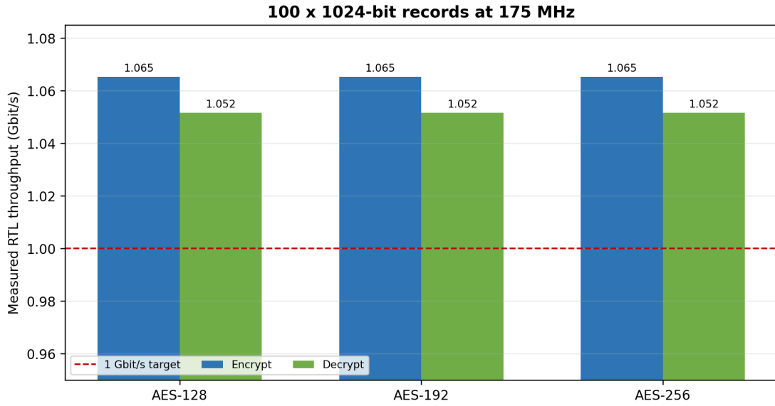
圖 4.1: 175 MHz 下的六模式 RTL throughput ; 三種 key size 皆大於 1 Gbit/s
