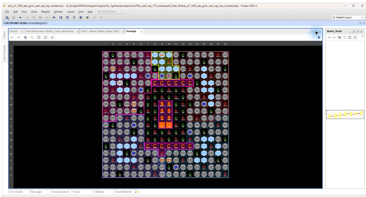
图 9.1: Vivado 原生 Package / I/O 视图；显示 XC7A100T CSG324 package、电源 / 时钟 / I/O pins 与 board-level pin planning。
